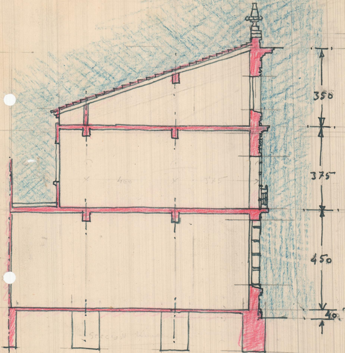
SECCION A-B
