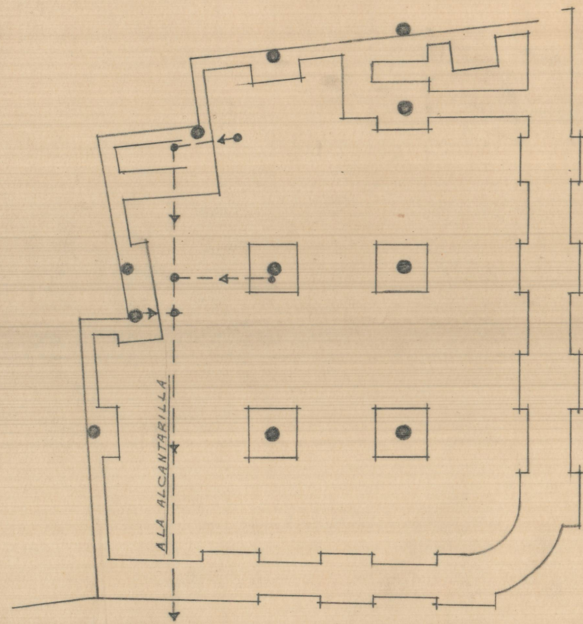
Planta de cimentación y de la vigas
