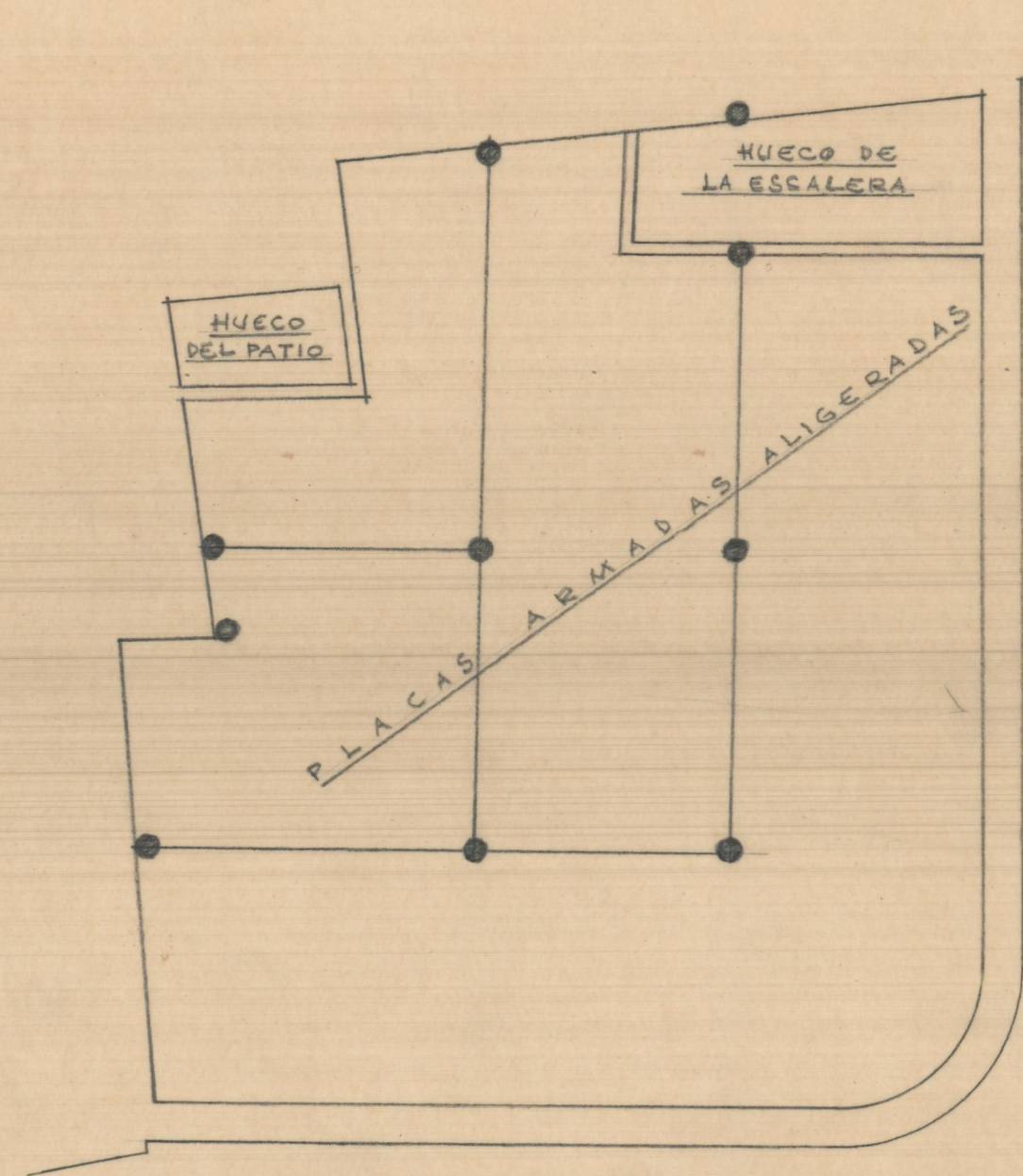
Planta entramado fijo de la segunda planta
