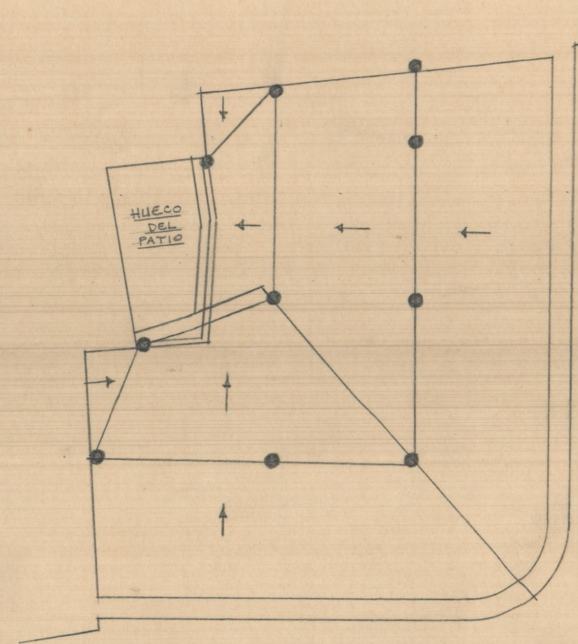
Planta de cubierta y placas armadas aligeradas
