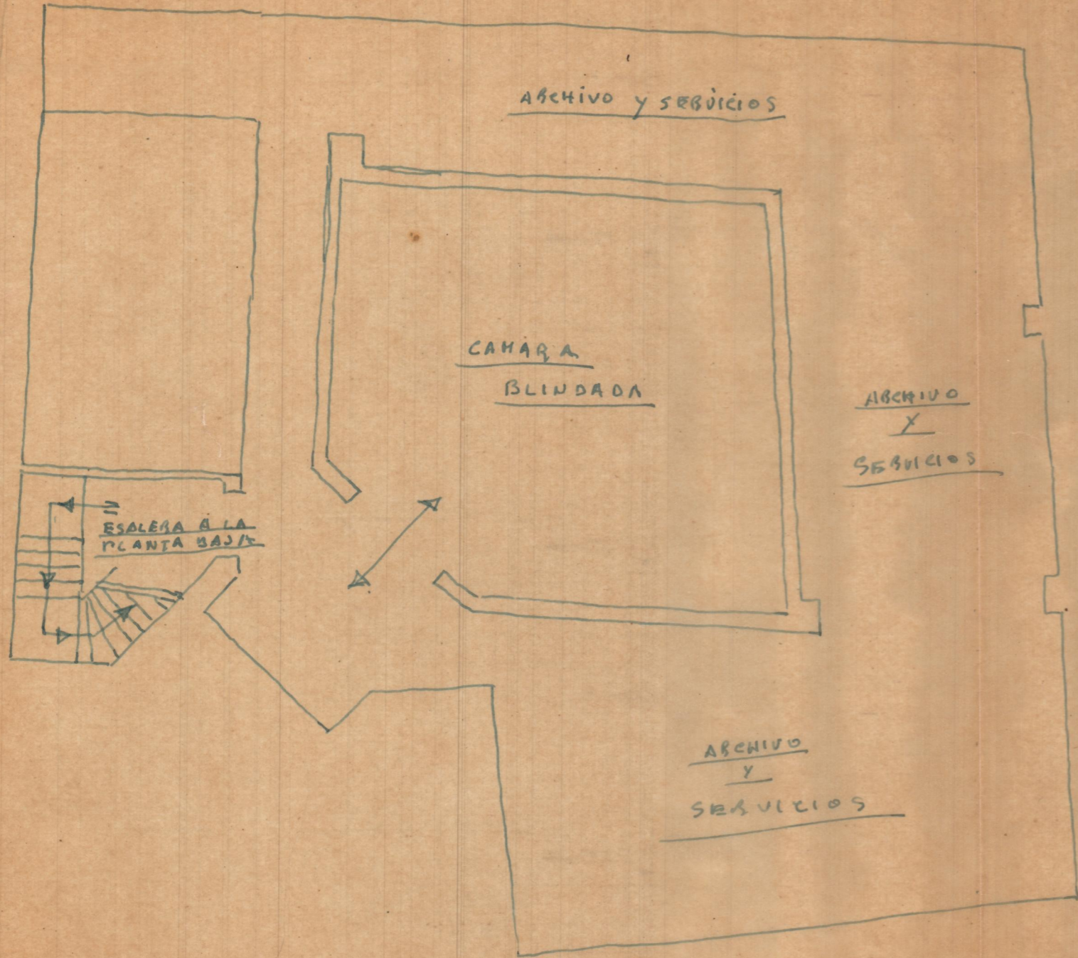
SOTANO - ESTADO ACTUAL
