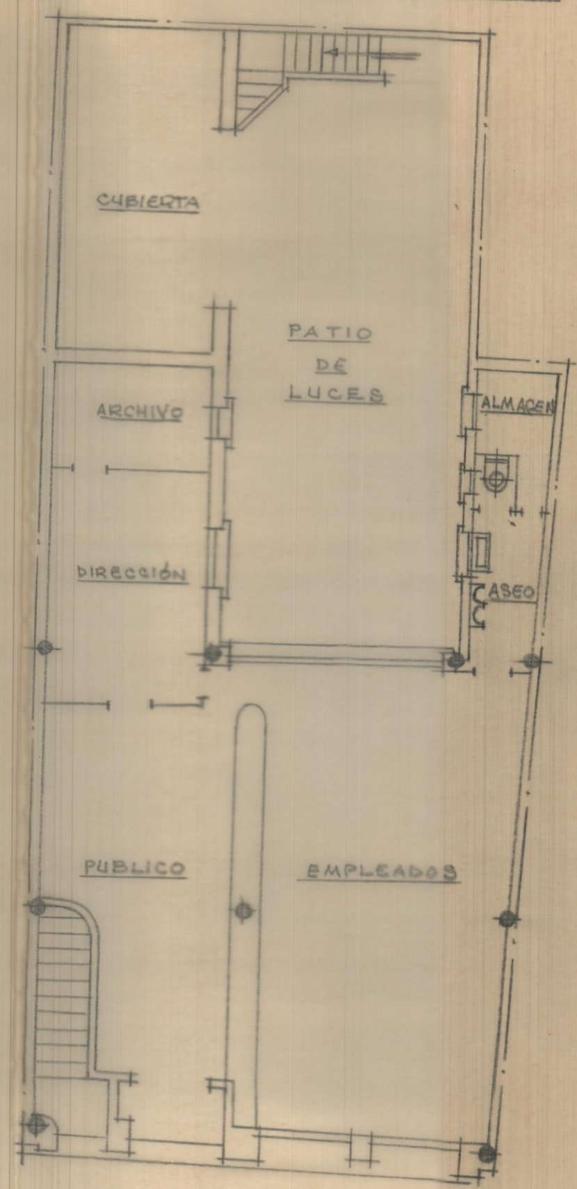
Planta baja
