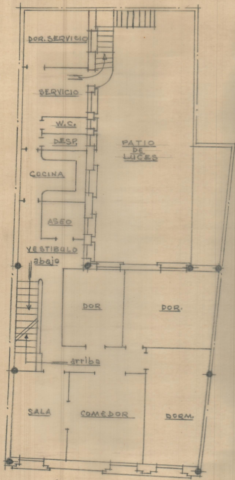
Planta alta
