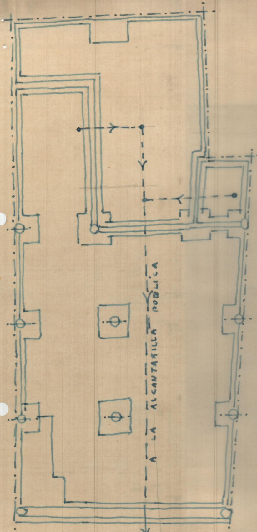
PLANTA DE CIMIENTOS Y DESAGUES
