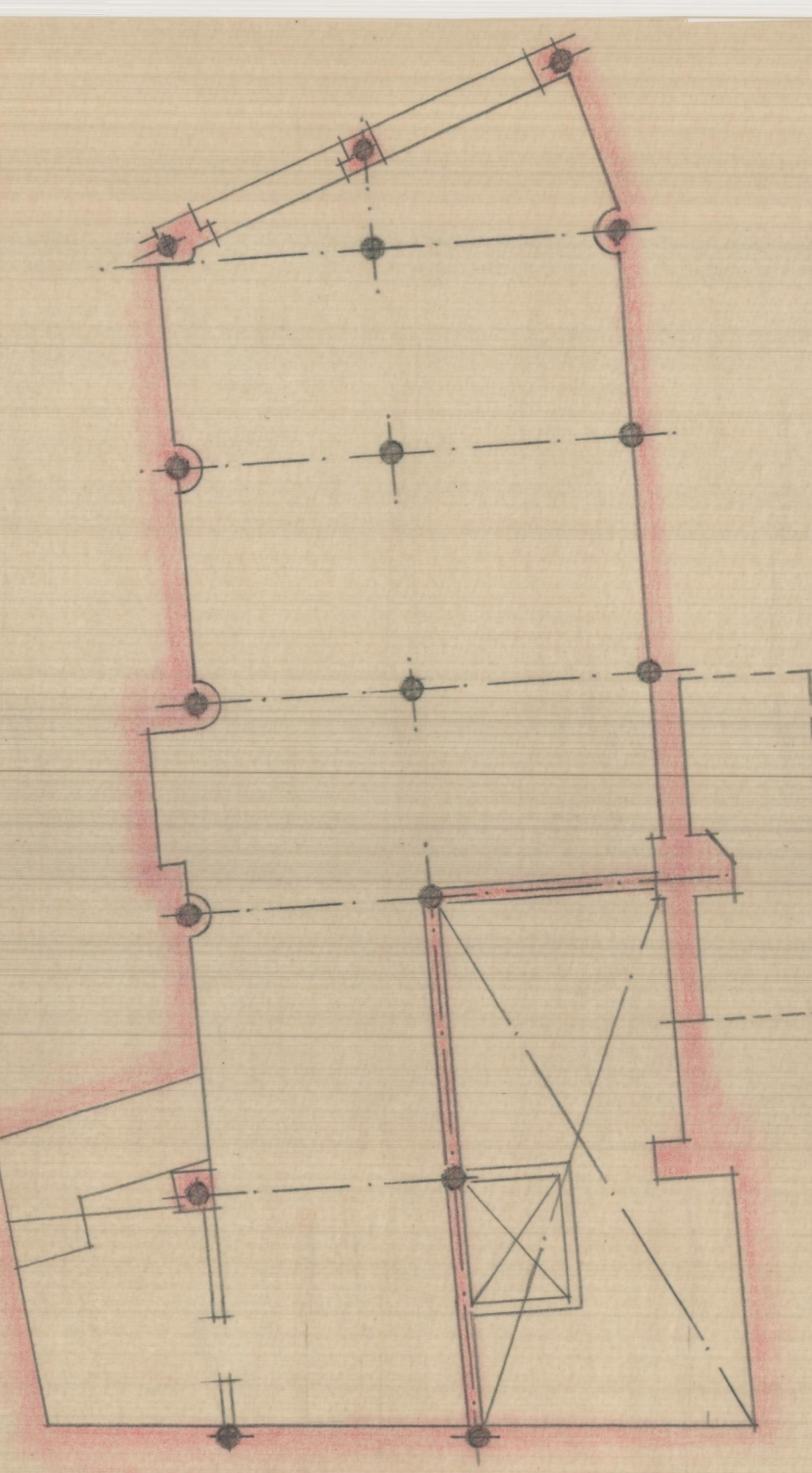
Pies y entramados piso alto
