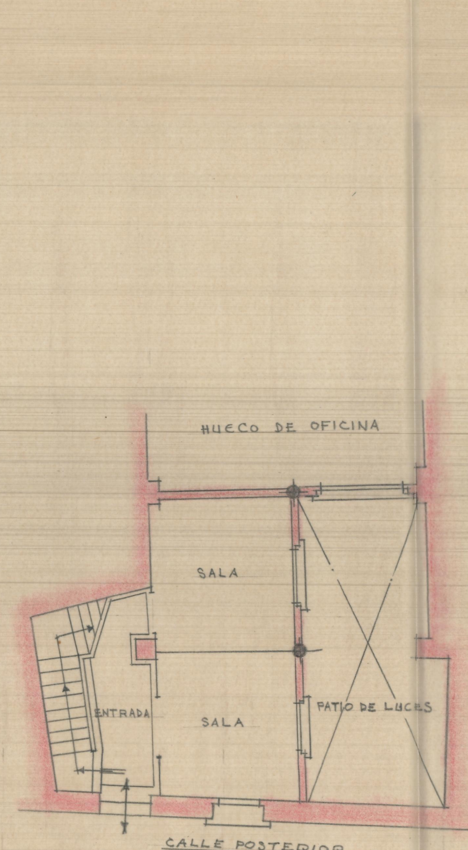
Entrepiso
