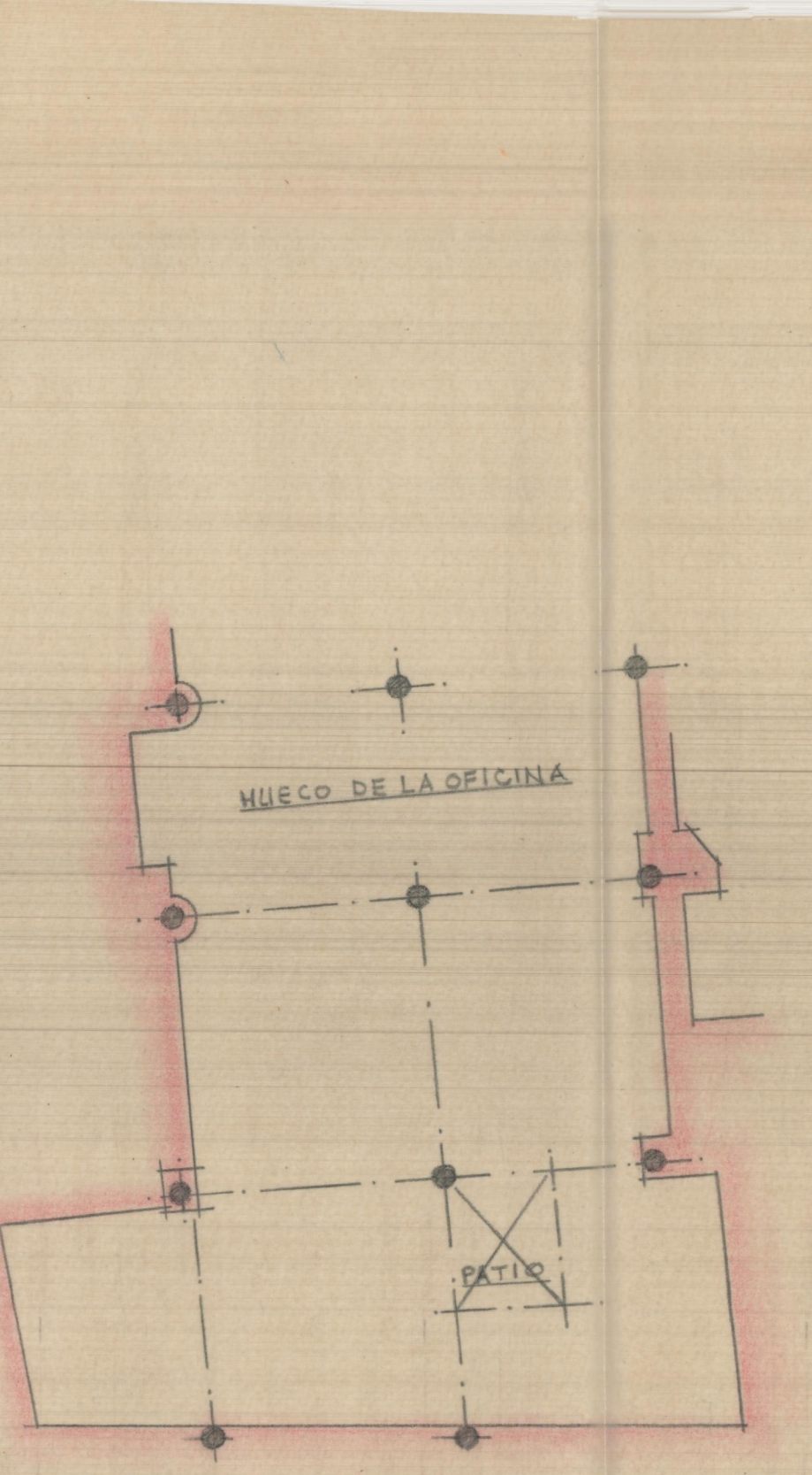
Pies y entramados del entrepiso
