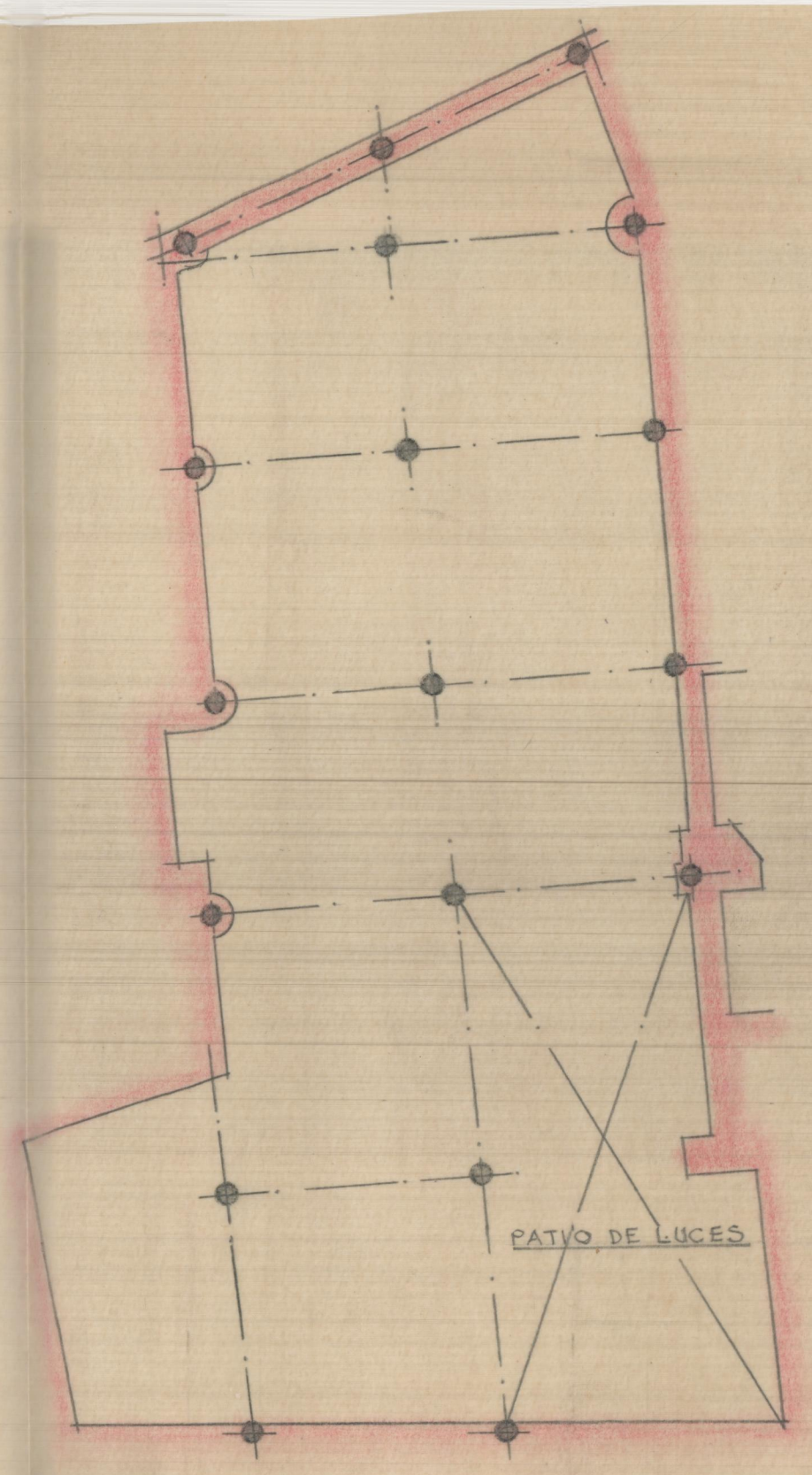
Pies y entramados de cubierta
