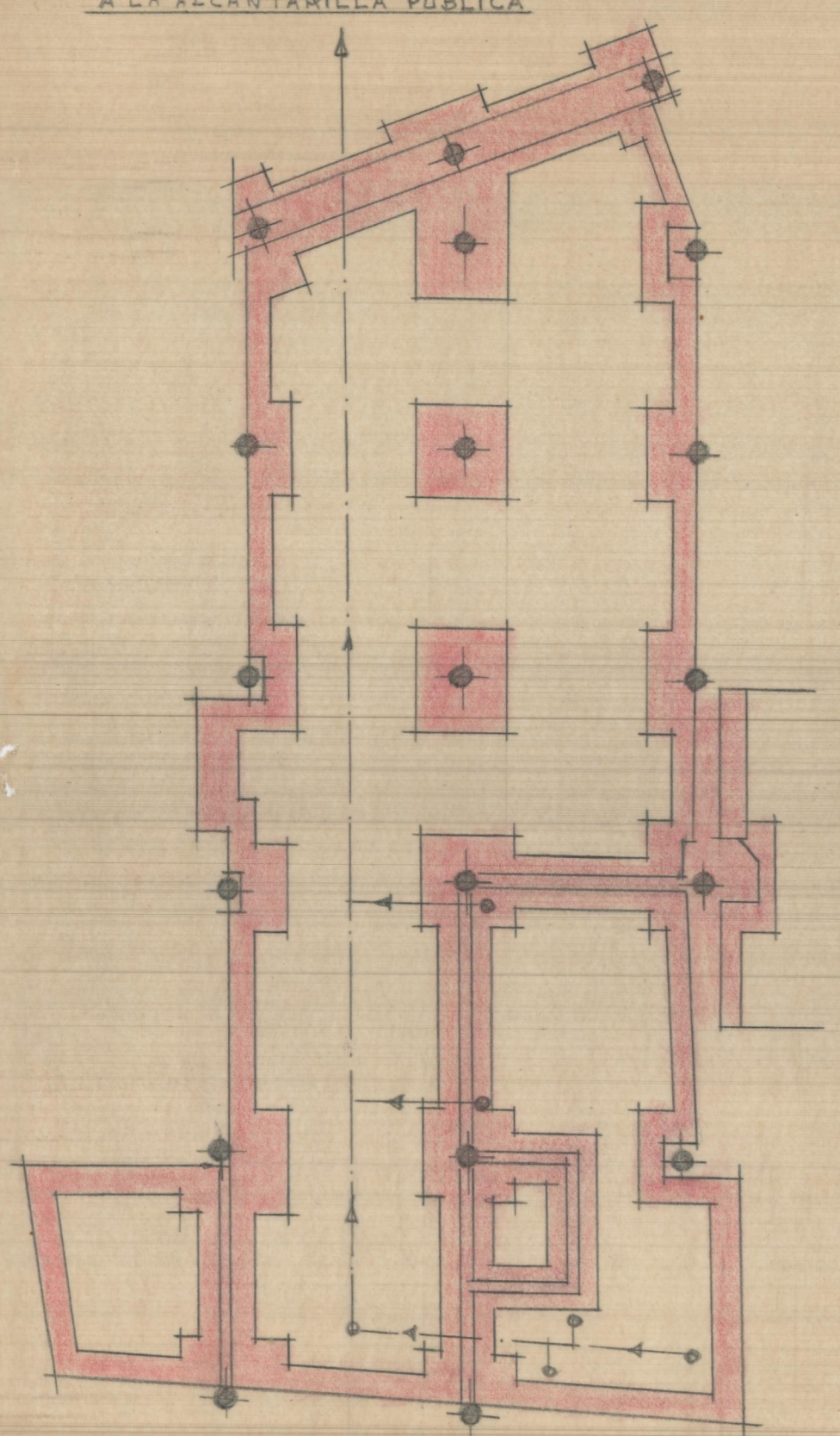
Cimientos y desagues
