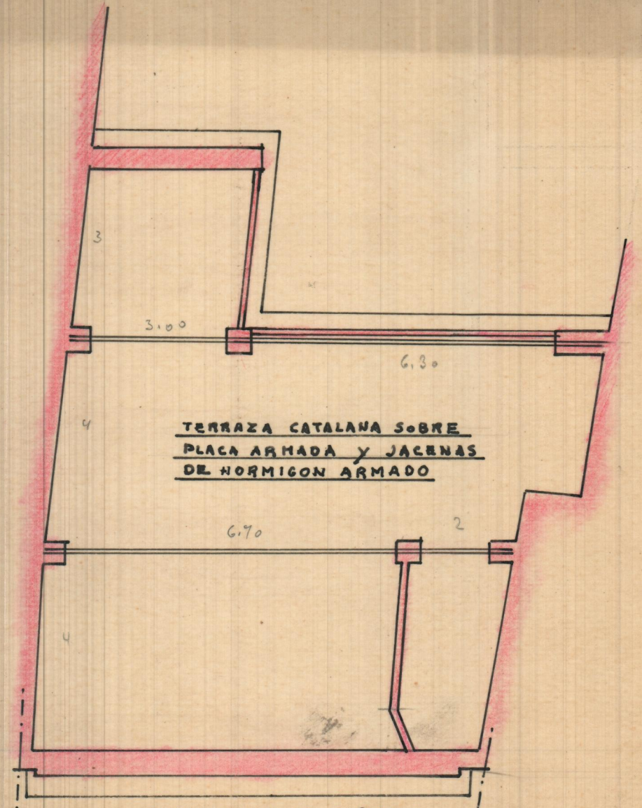
ESTRUCTURA DE CUBIERTA
