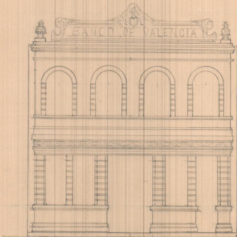
Fachada
