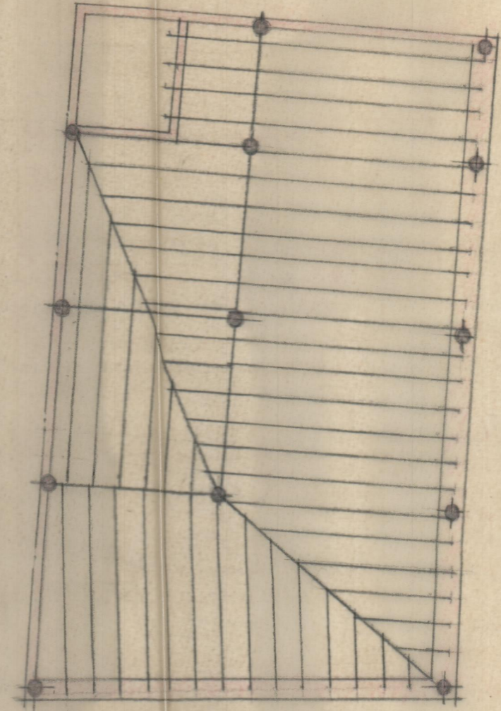
Entramado cubierta
