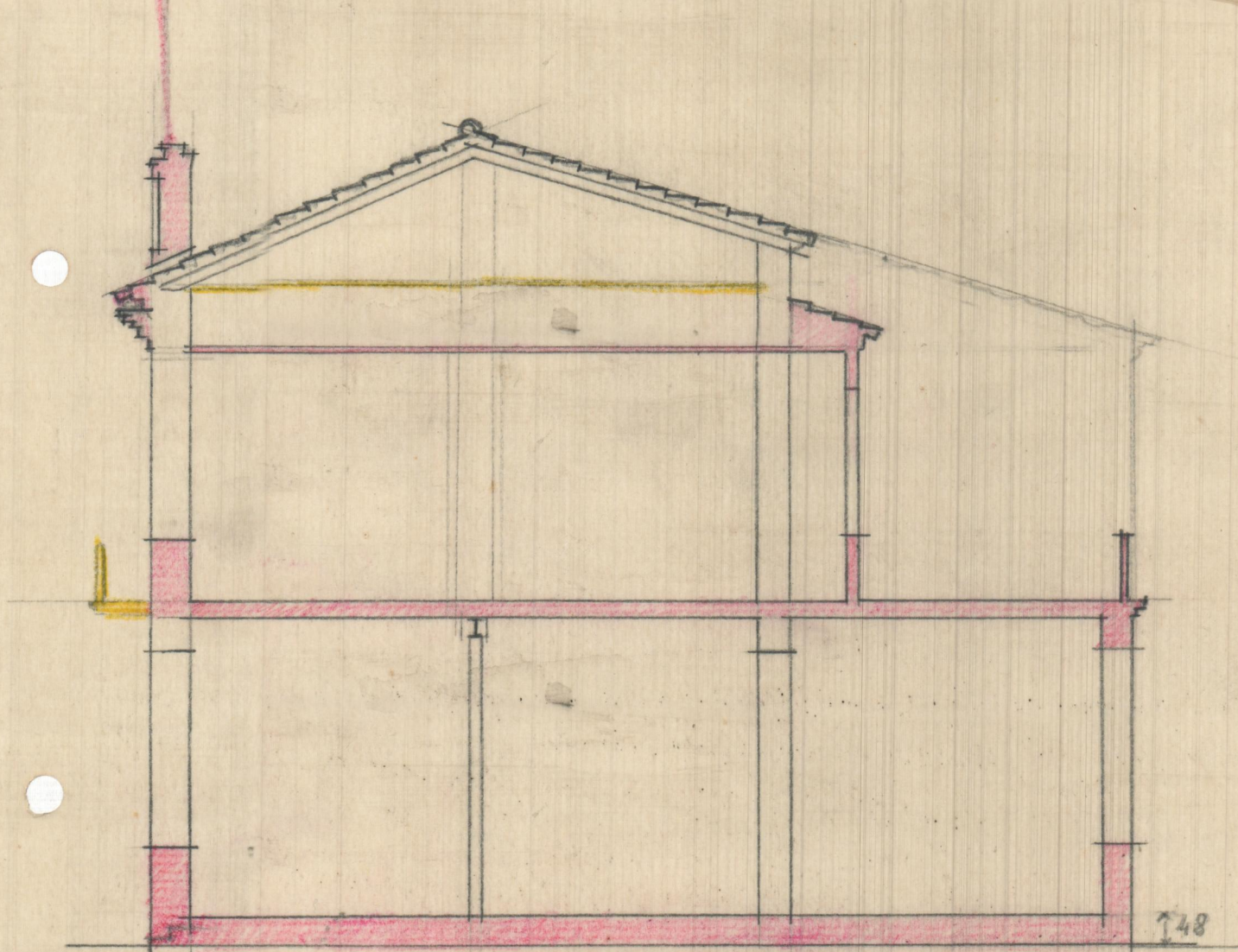
SECCION LONGITUDINAL
