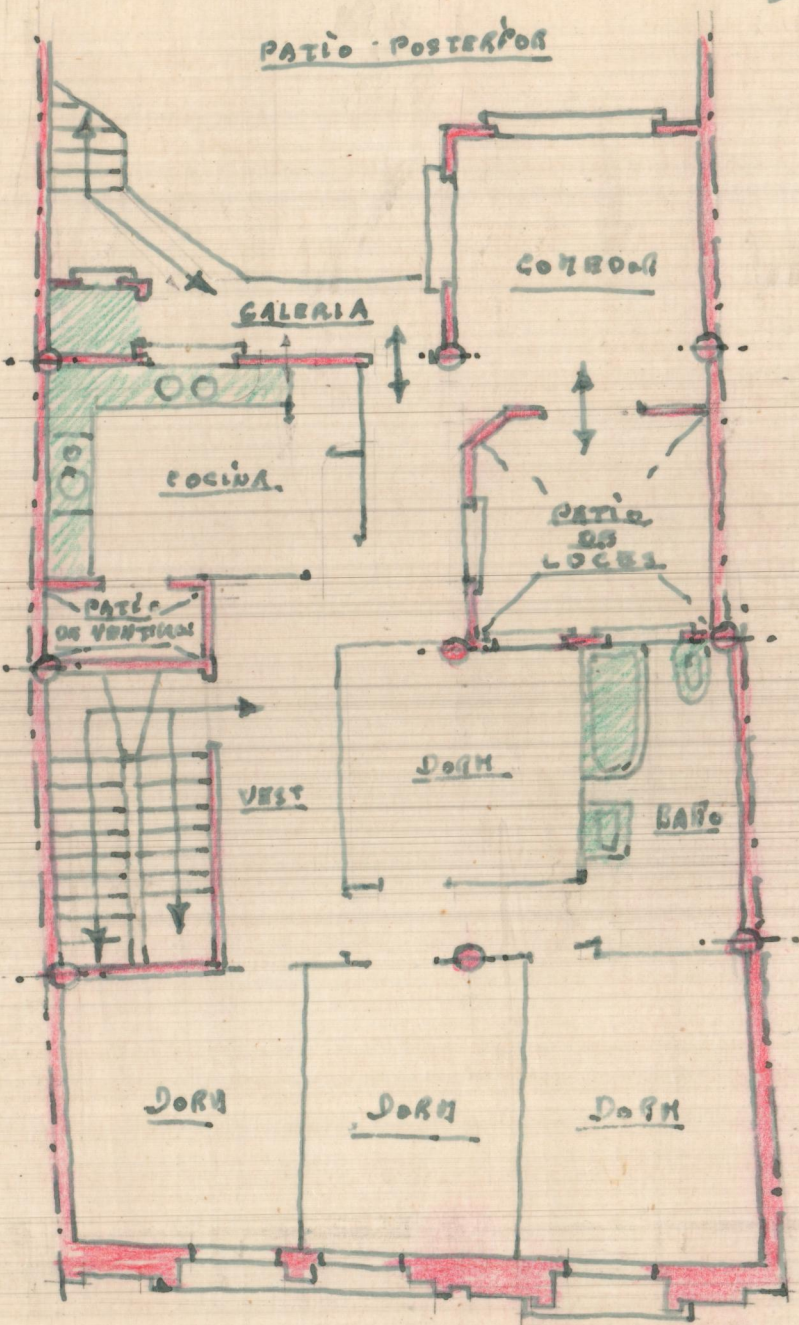
NUEVA DISPOSICION DE PATIOS DE LUZ Y VENTILACION
