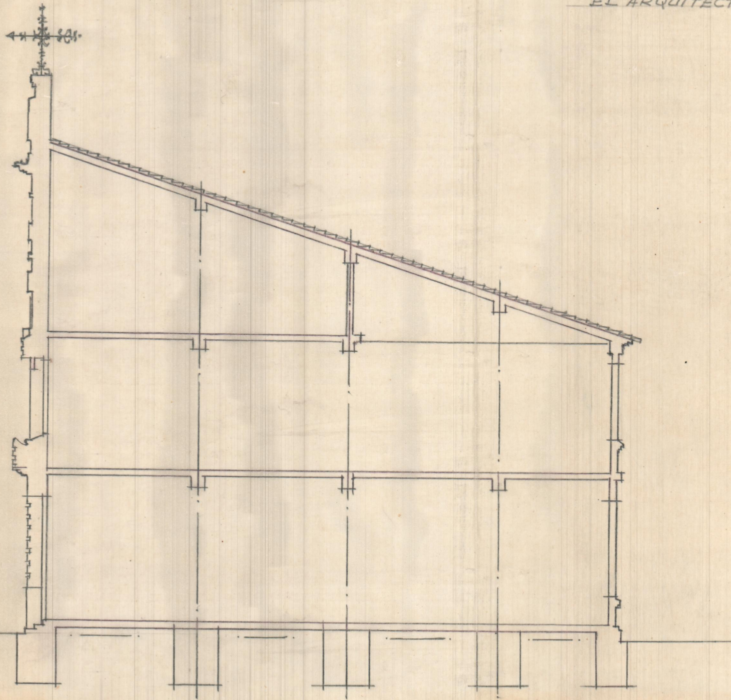
Sección A-B.
