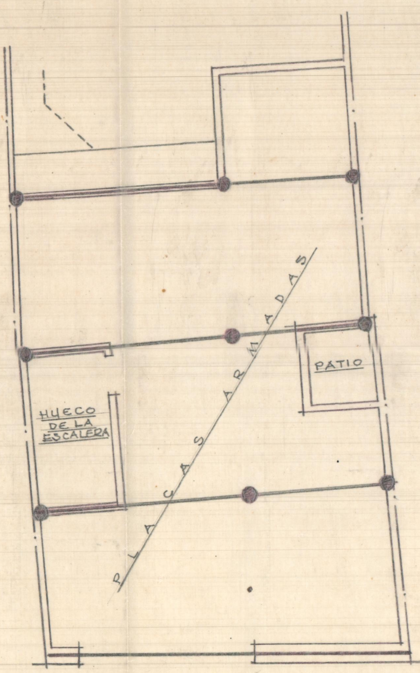
Entramado del piso primero.
