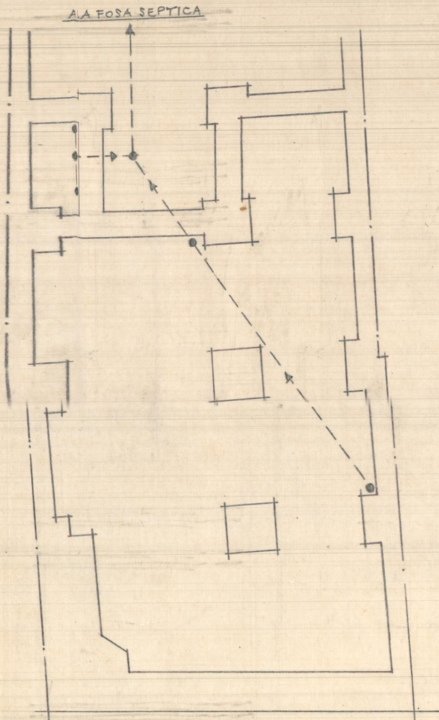
Planta de cimientos y de columnas
