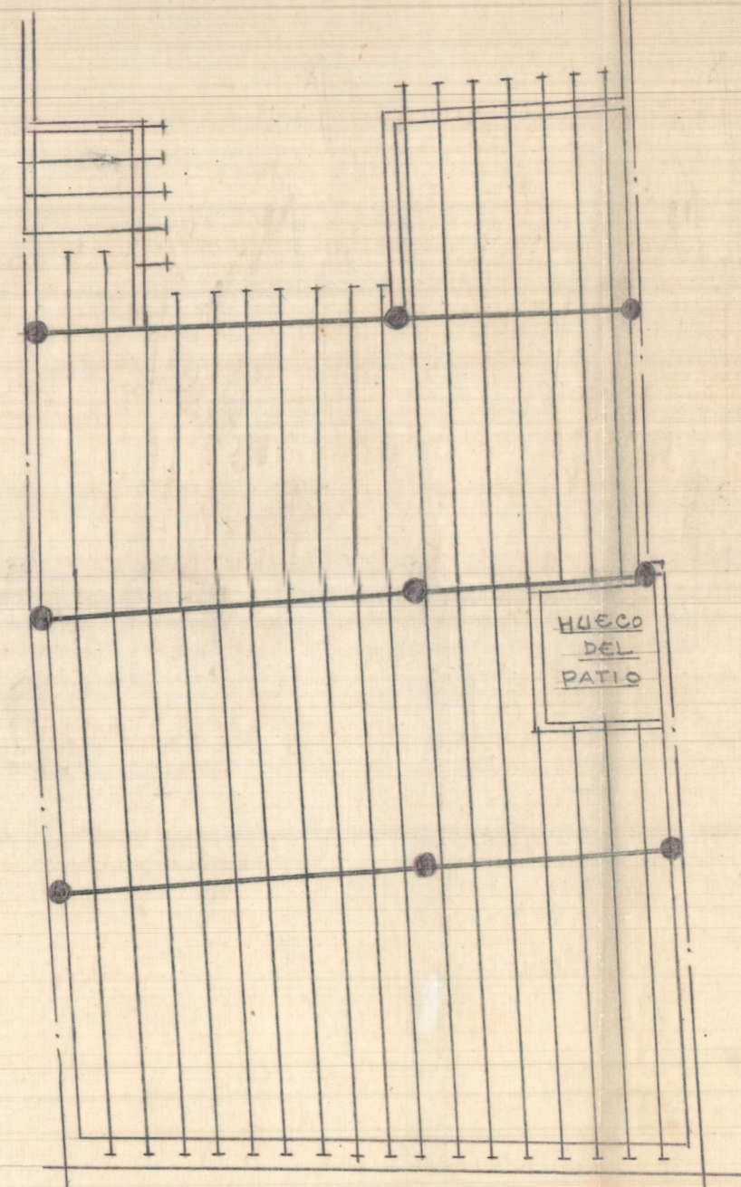
Entramado de cubierta
