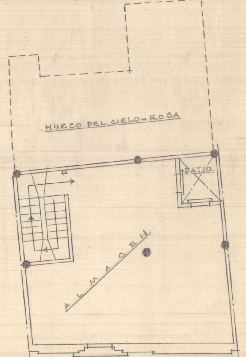
Disposicion de la ultima planta
