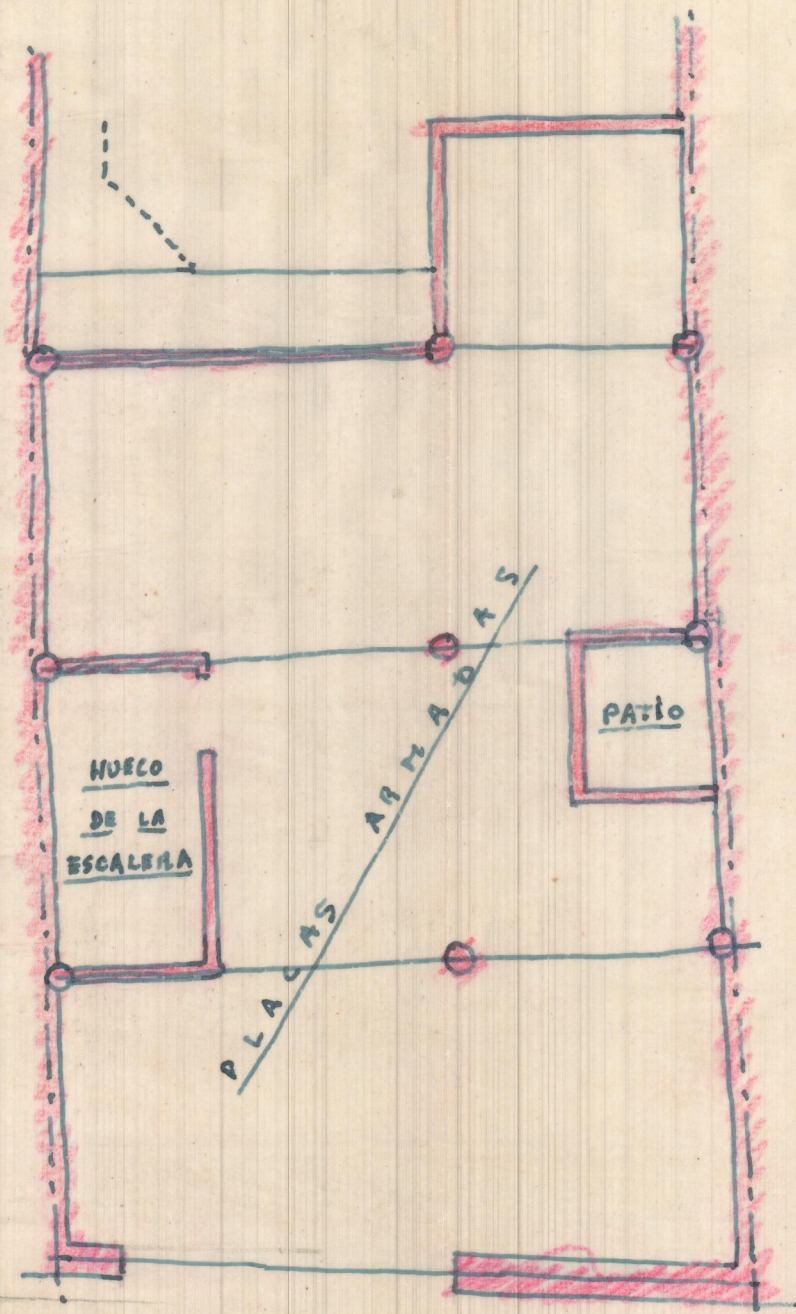
ENTRAMADO DEL PISO PRIMERO
