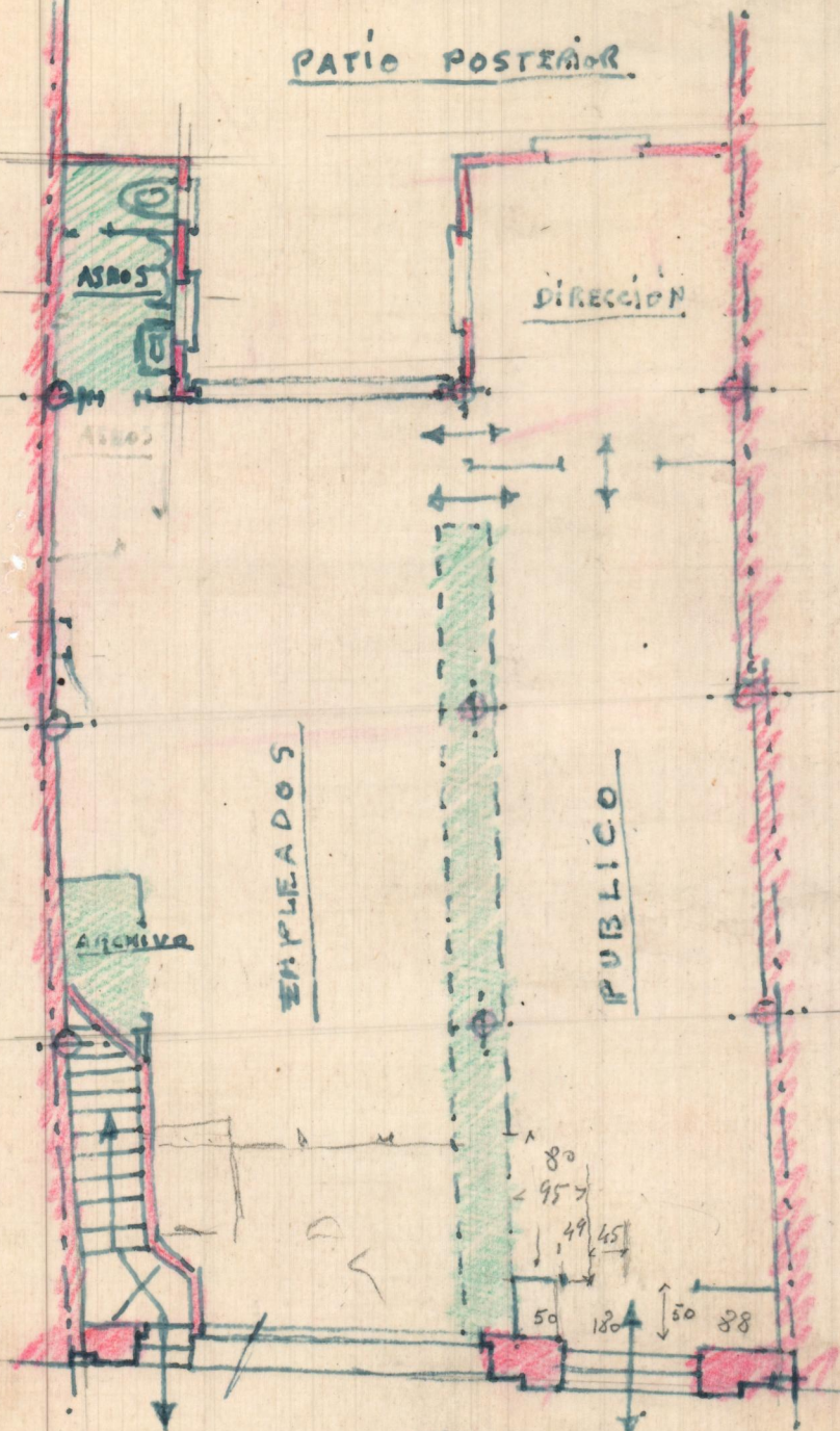
OFICINAS-DISPOSICION
