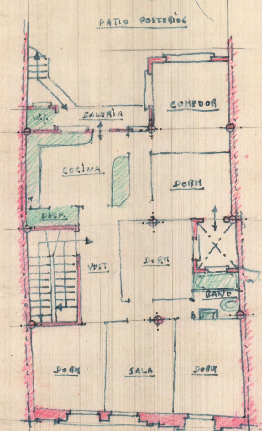
DISPOSICION DE LA VIVIENDA VARIANTE
