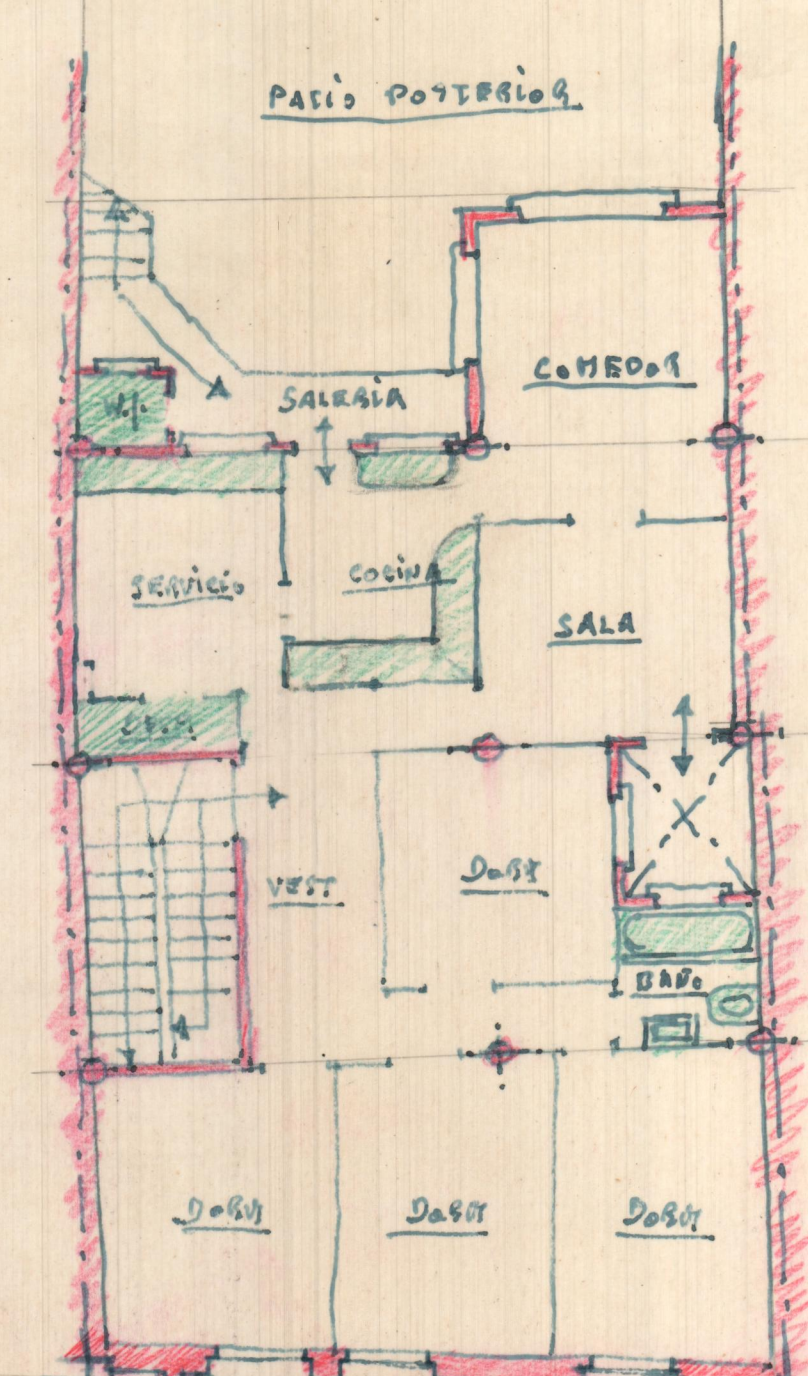
DISPOSICION DE LA VIVIENDA
