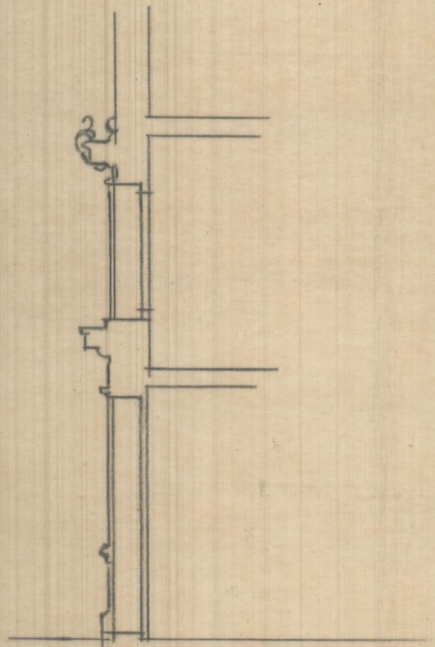
Sección vertical
