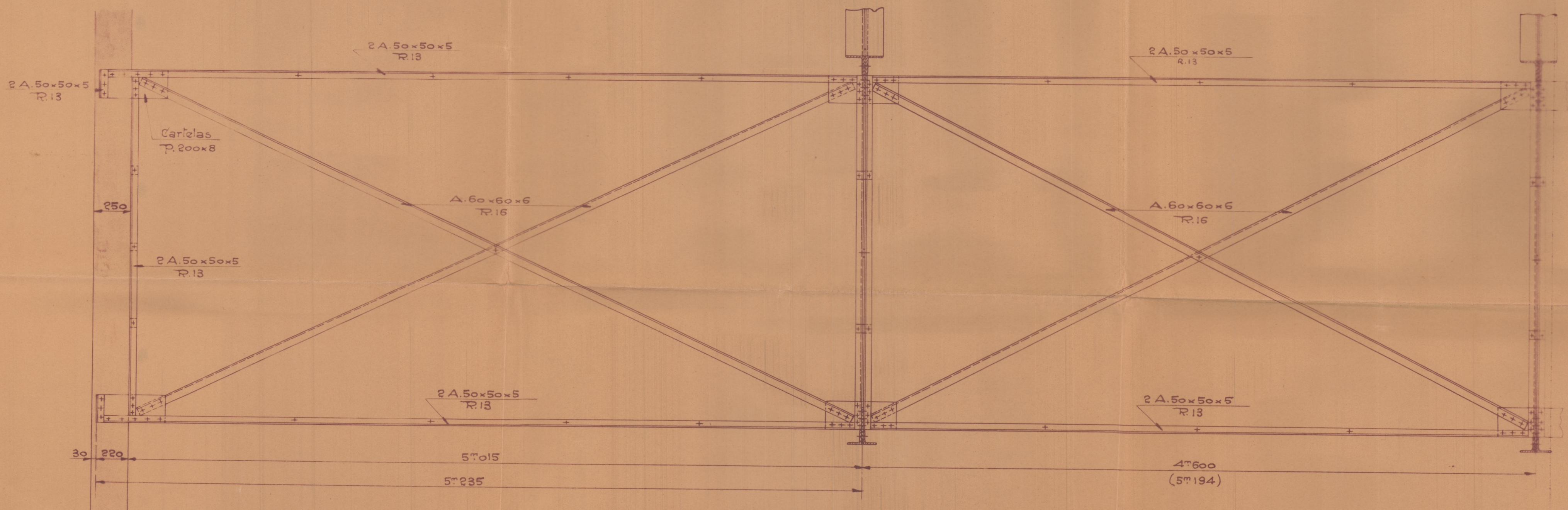
Arriostrado entre cuchillos HH'GG' y FF'(4" 600) y entre cuchillos FF'EE' y DD'(5" 194)
