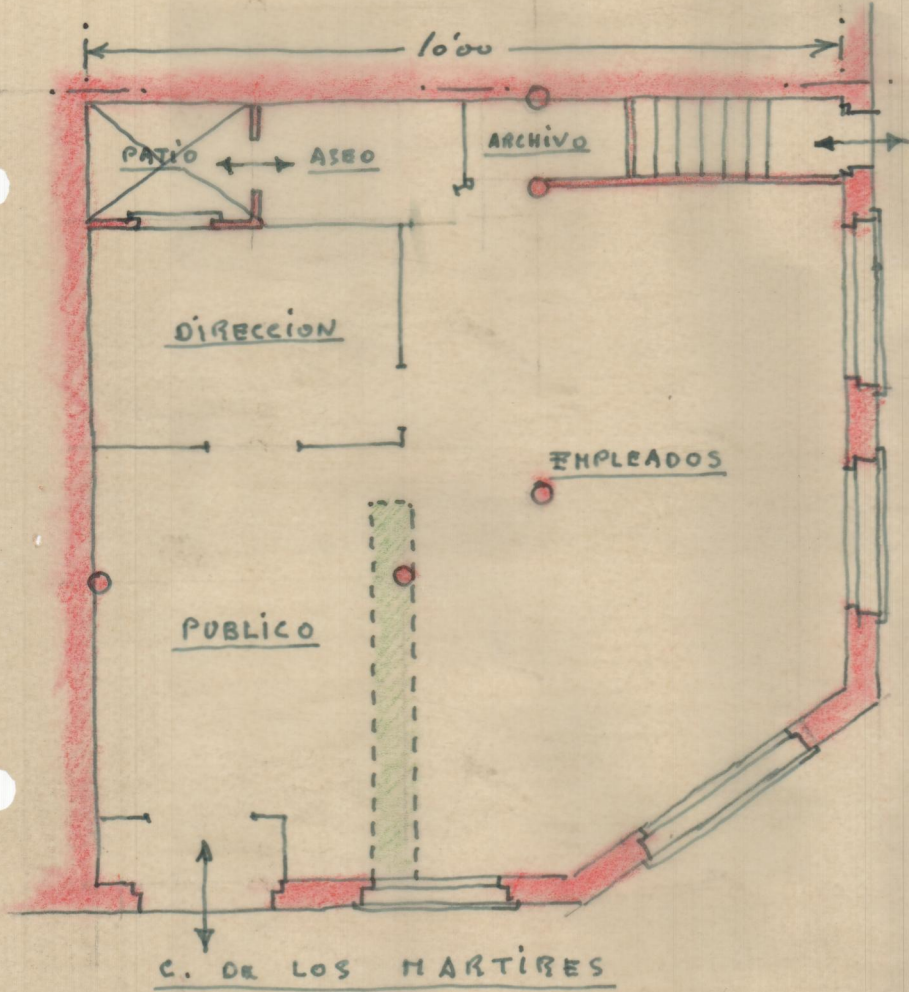
PLANTA BAJA
