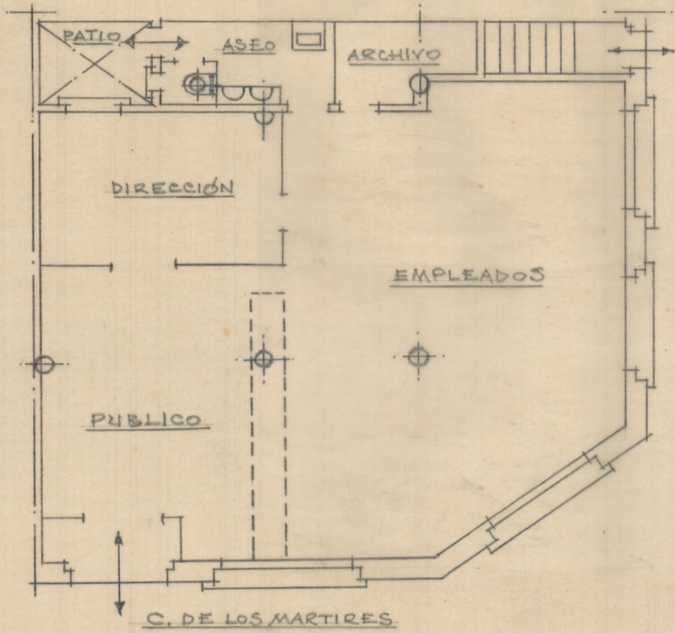
Planta baja
