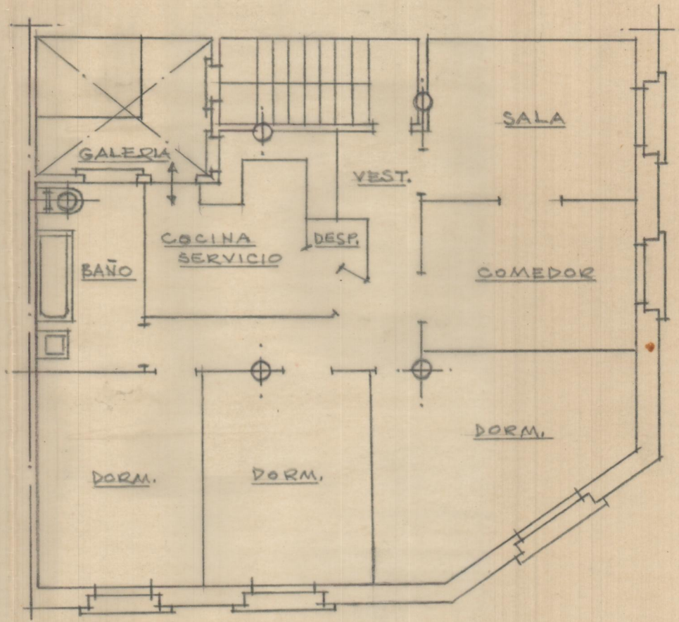
Piso - vivienda
