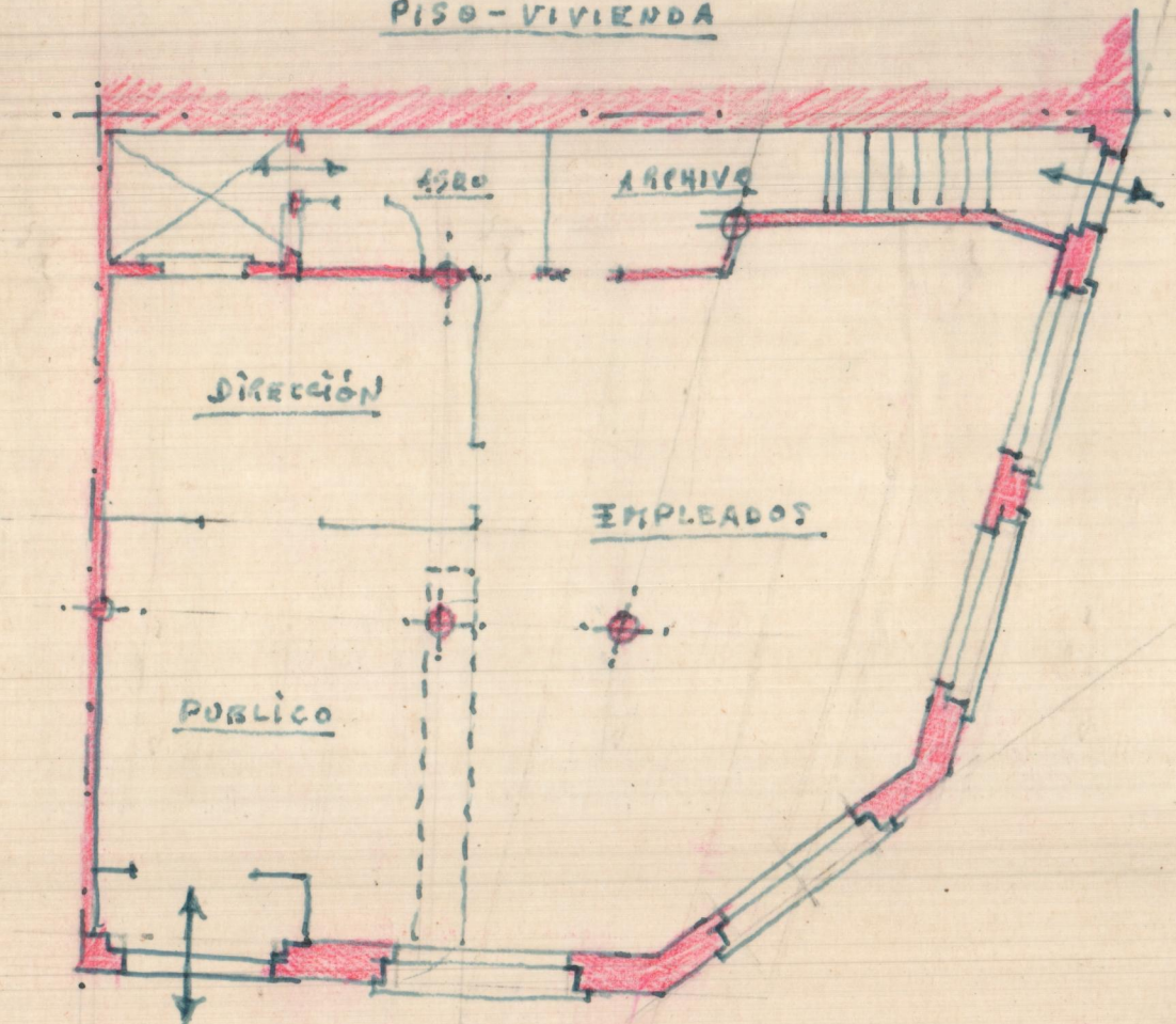
PLANTA BAJA
