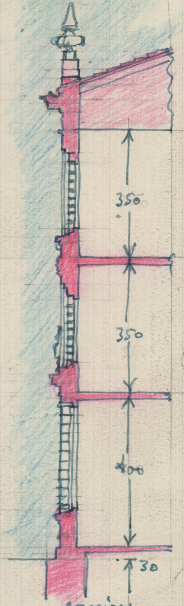
SECCION
