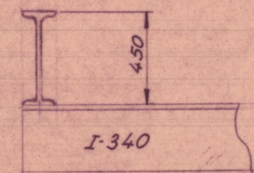
Detalle W
