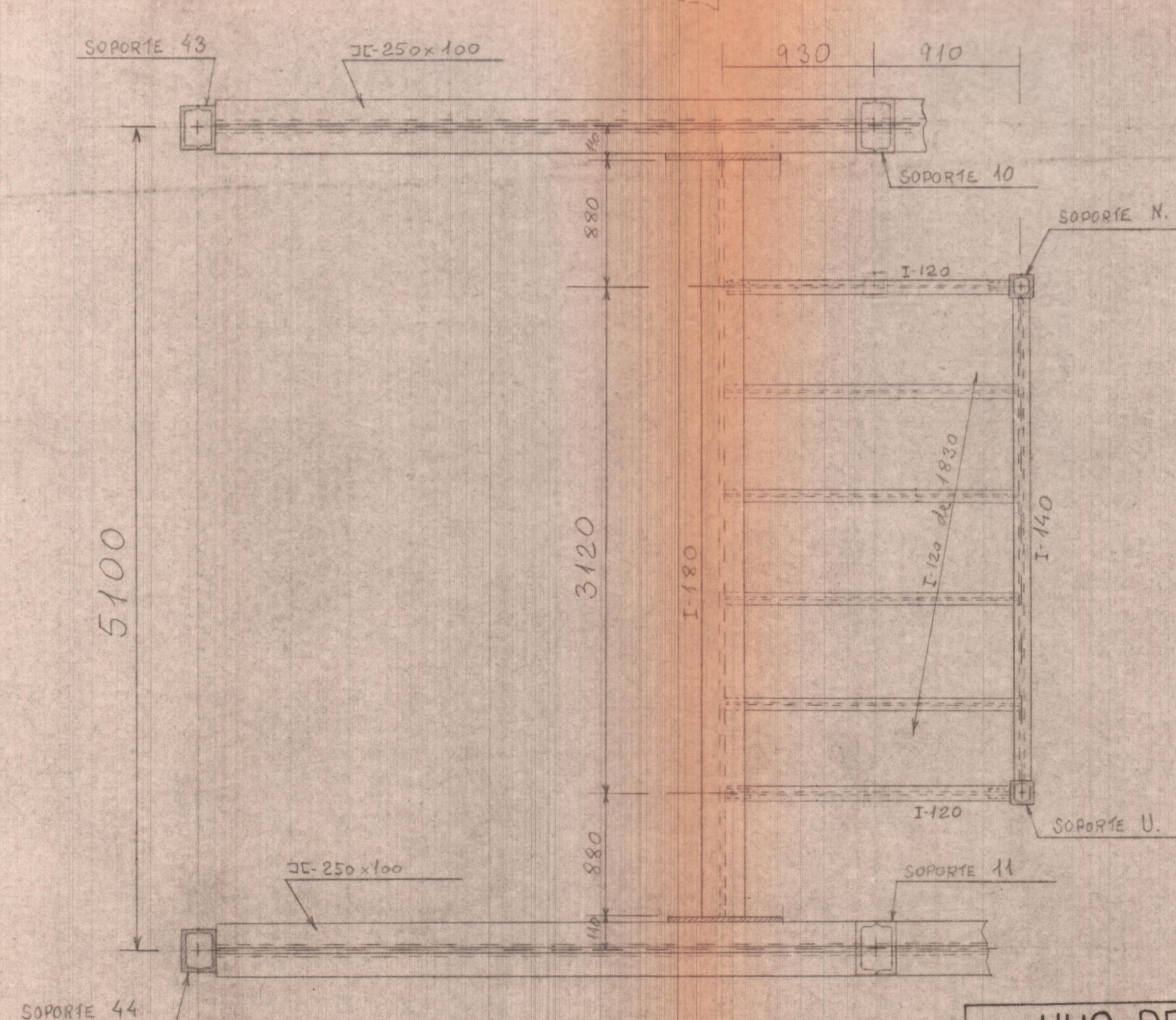
PLANTA PALCO EN GRADERIO
