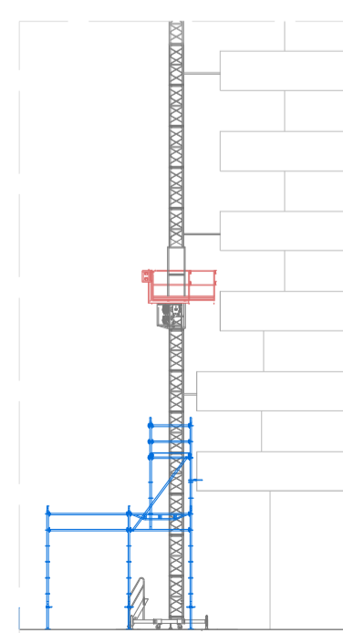
PERFIL
