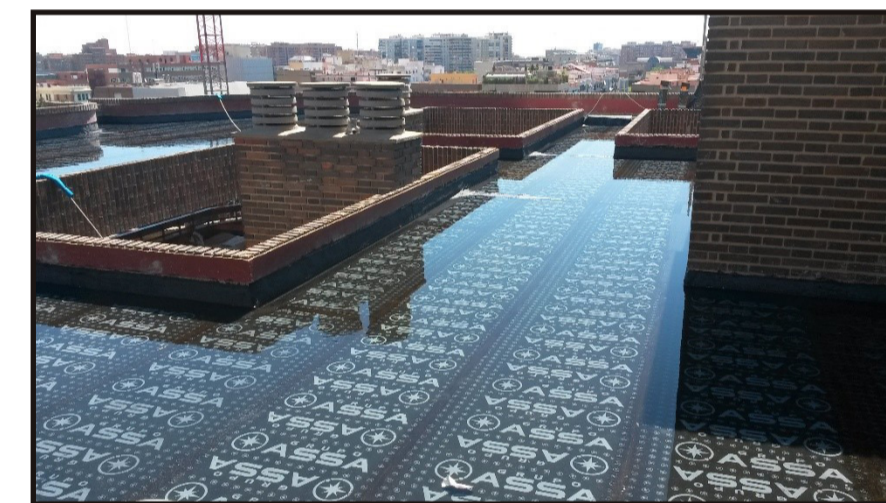
Pruebas de estanqueidad en cubiertas.
