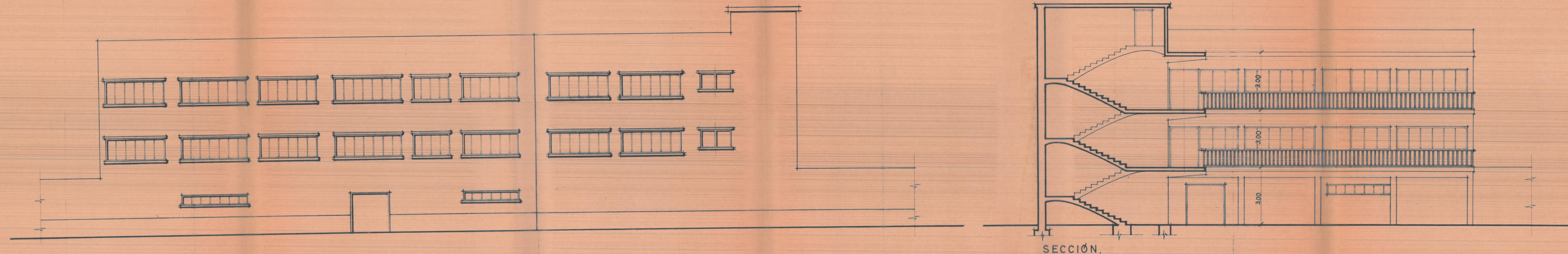
ALZADOS. (desarrollo.)
