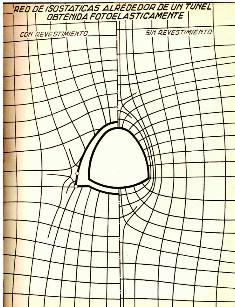
Figura 8. Red de isostáticas alrededor de un túnel obtenida fotoelásticamente. Fuente: R.O.P. Nº extraordinario dedicado al cincuentenario del Laboratorio Central..
