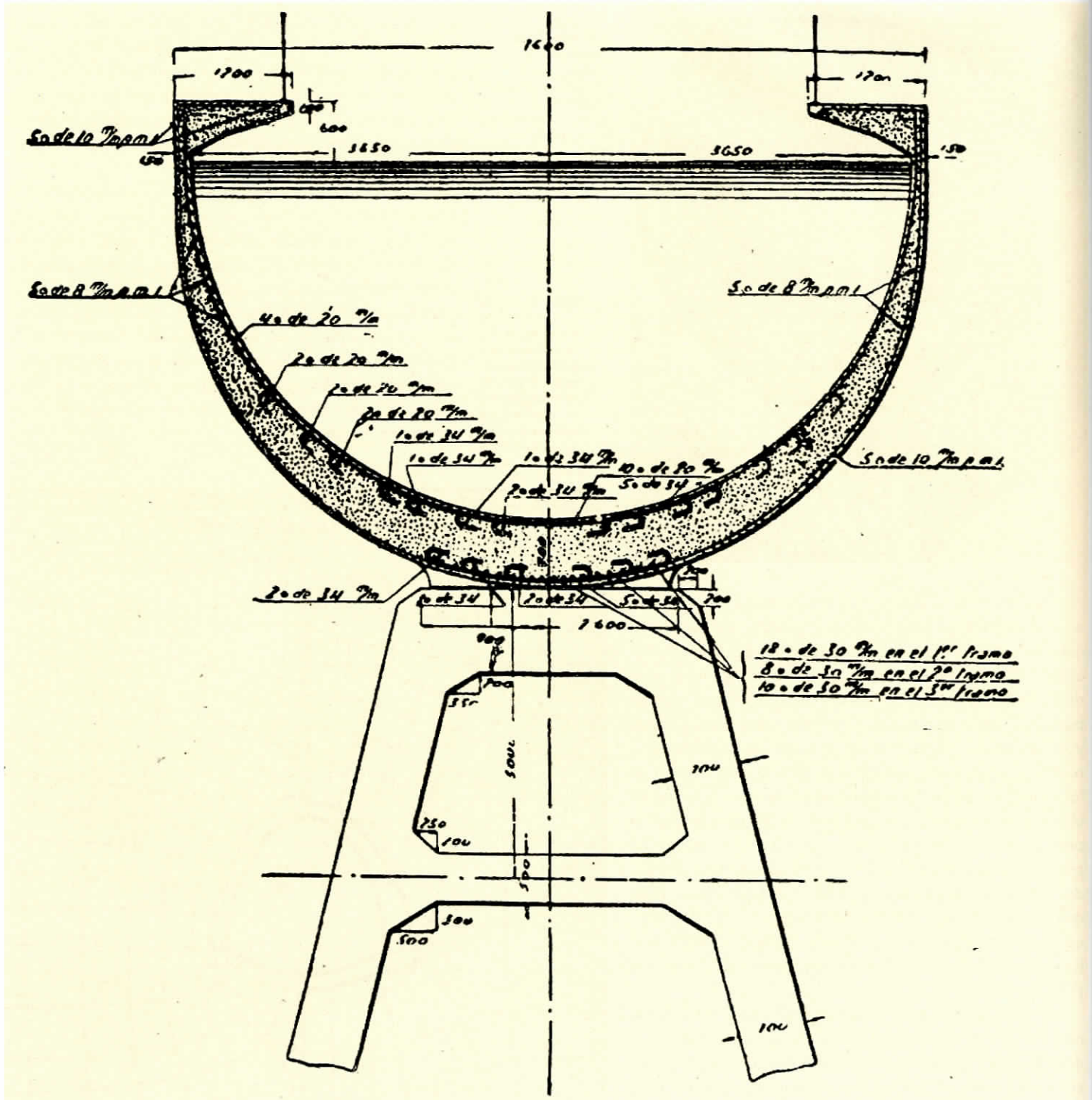
Figura 9. Acueducto de Tardienta. Sección transversal. Fuente: R.O.P. 1941.
