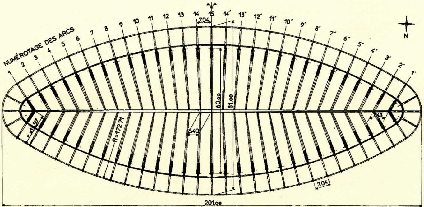
Fig. 4. a — Plano de conjunto de la cubierta.
