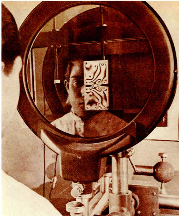
Figura 7. Laboratorio de fotoelasticidad. Fuente: R.O.P. Nº extraordinario dedicado al cincuentenario del Laboratorio Central.
