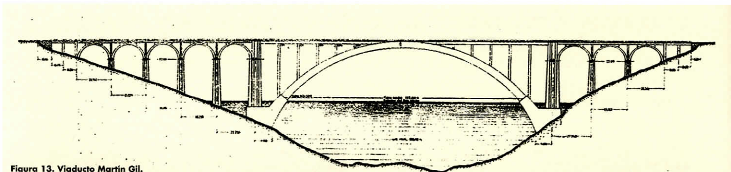
Figura 13. Viaducto Martín Gil. Fuente: R.O.P. 1942.
