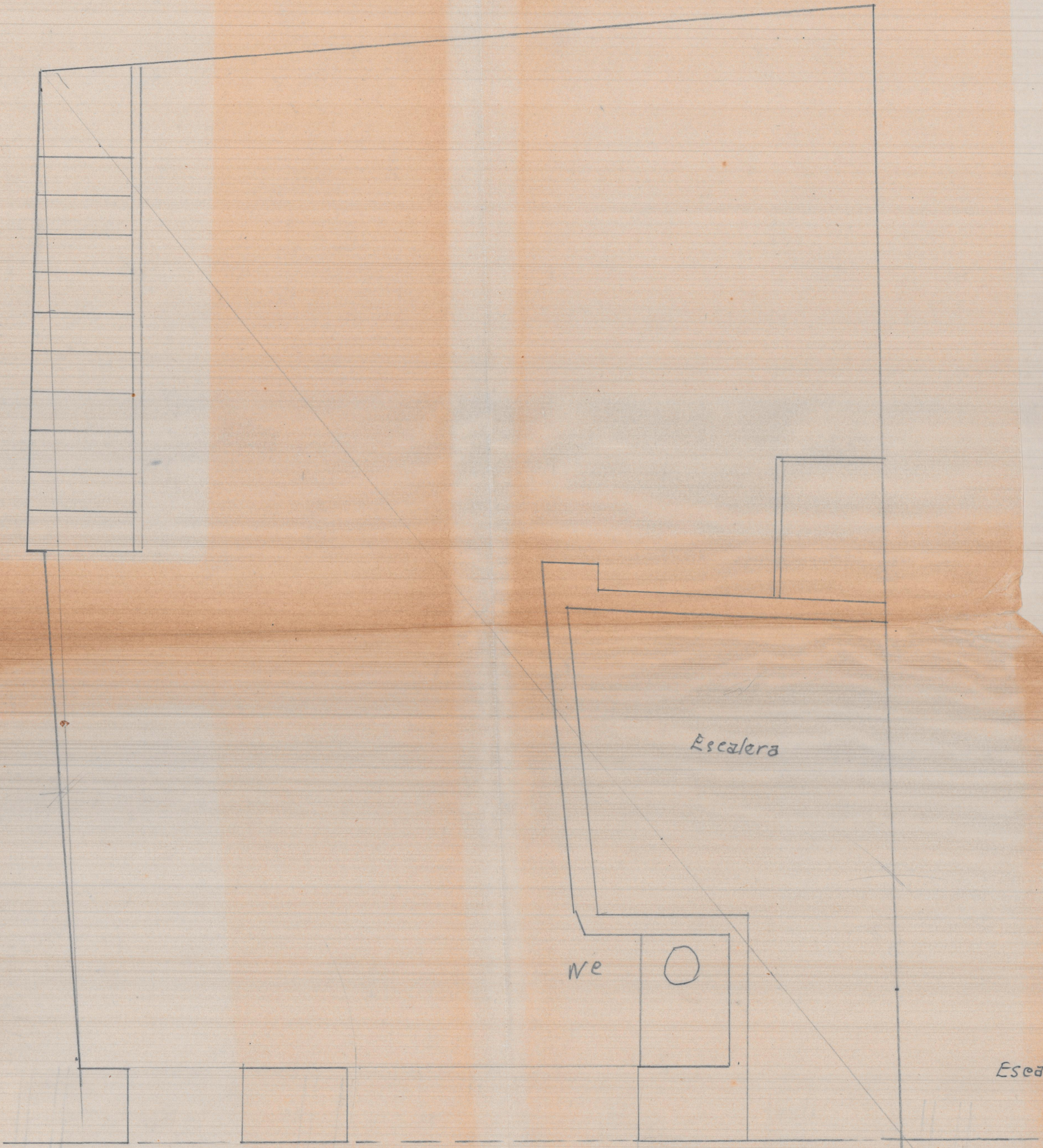
Casa n°8 del Portillo de San Jorge - Planta
