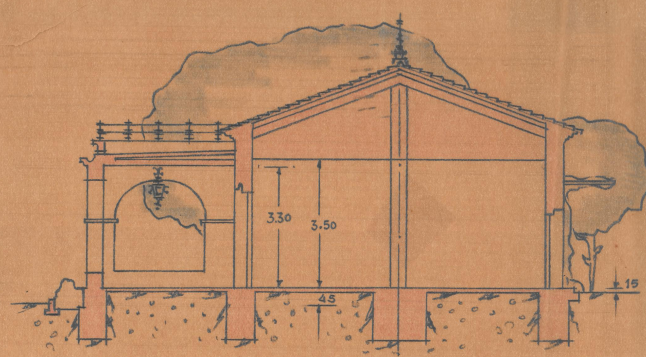
Sección longitudinal
