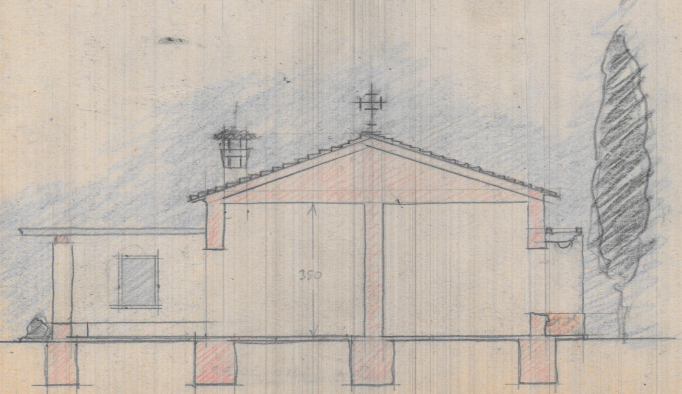
SECCION A-B
