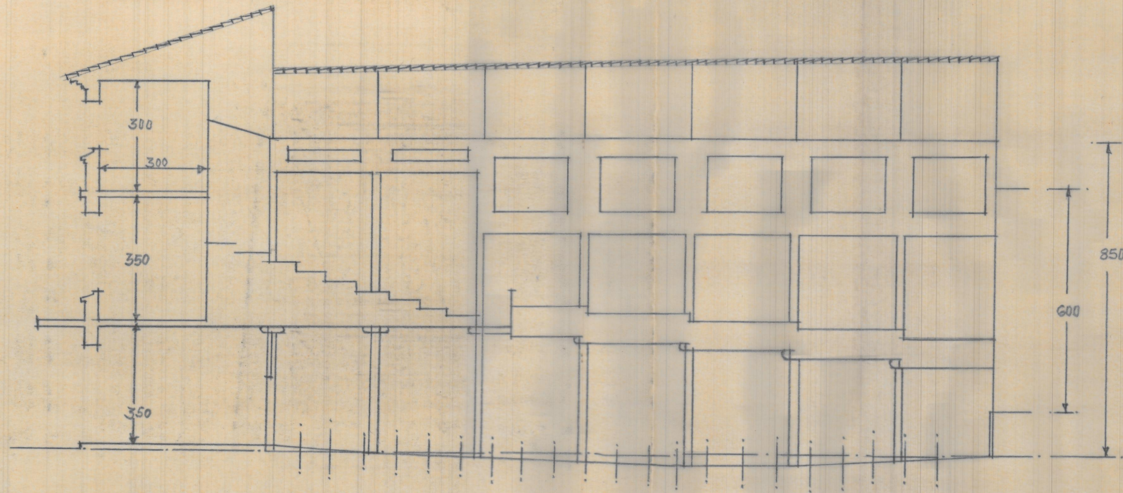
Sección por A.B.
