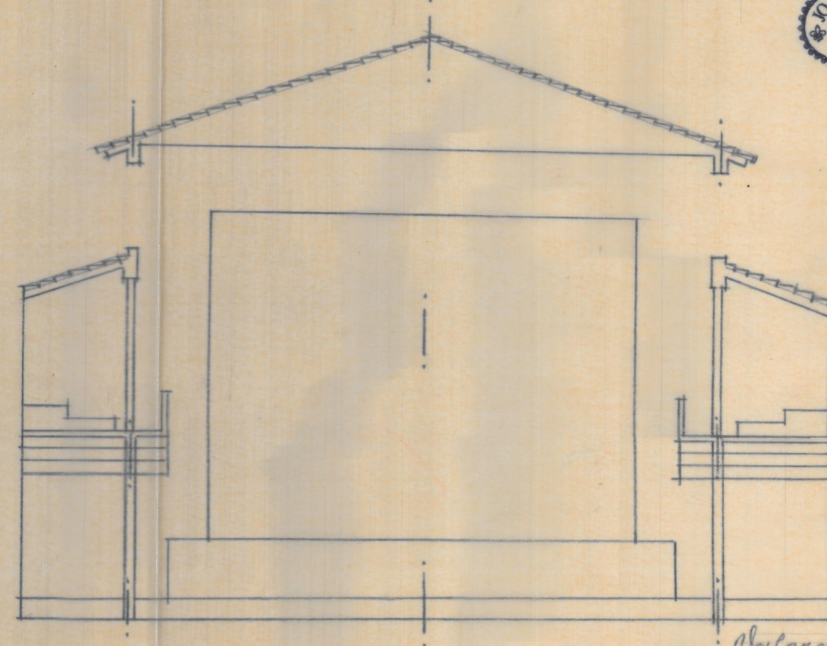
Sección por C.D.
