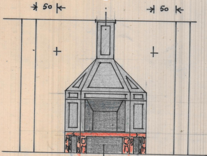
FRENTE
