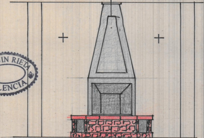
FRENTE
