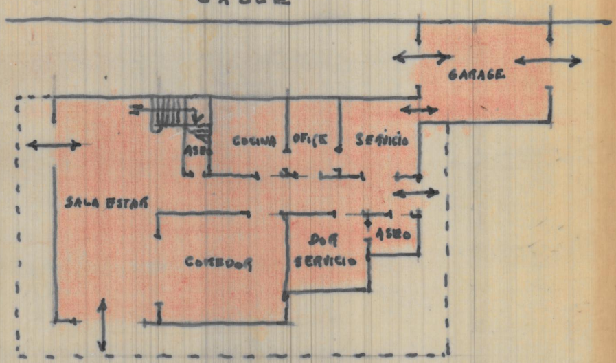
PLANTA BAJA
