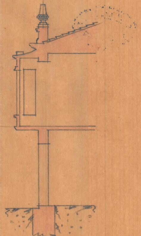
Sección A-B
