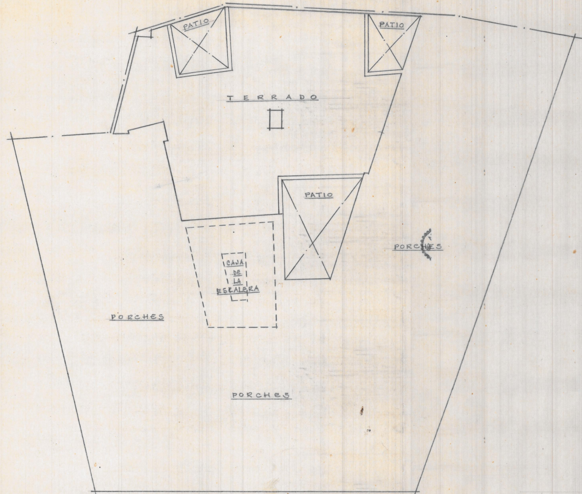
Disposicion actual de la ultima planta
