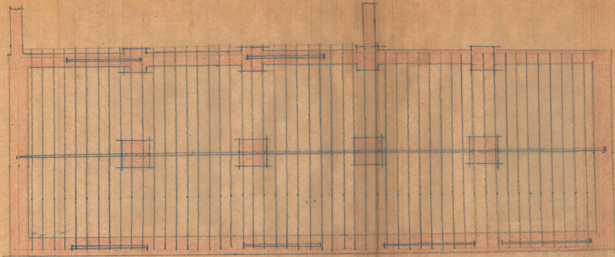
PLANTA DE CIMIENTOS Y ENTRAMADOS
