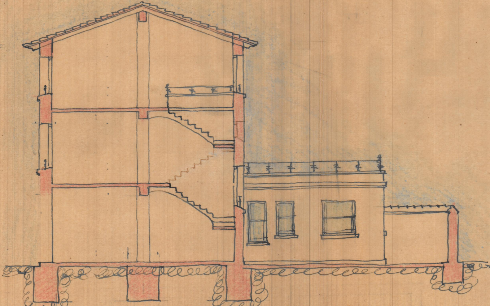
SECCION LONGITUDINAL
