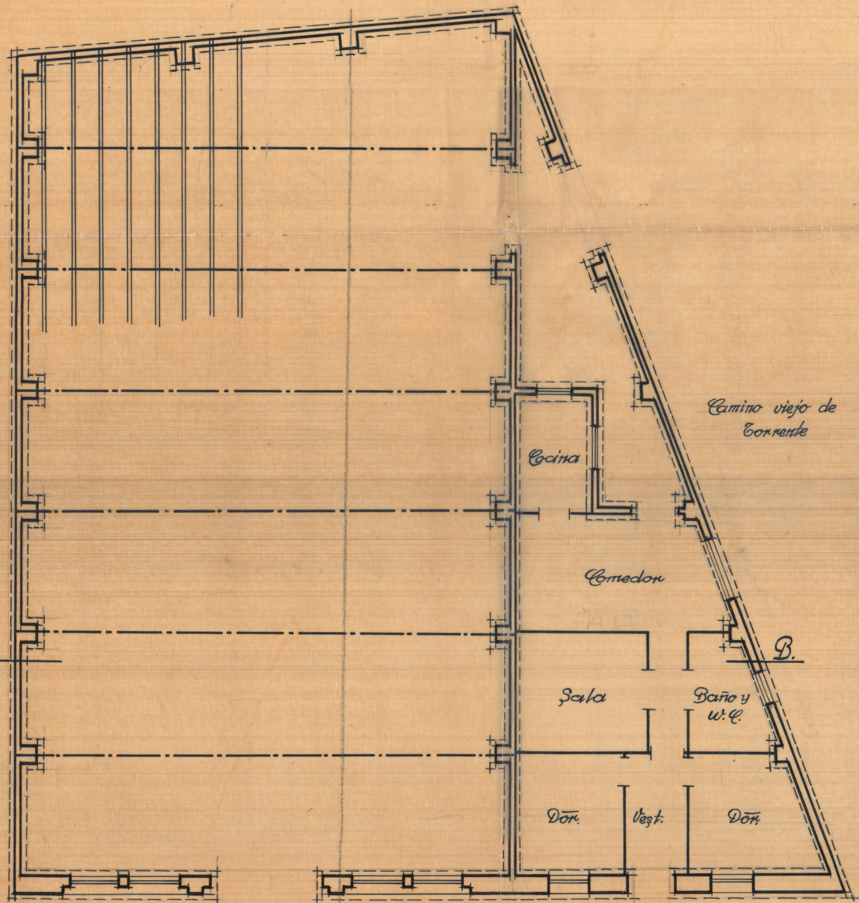
Plantas
