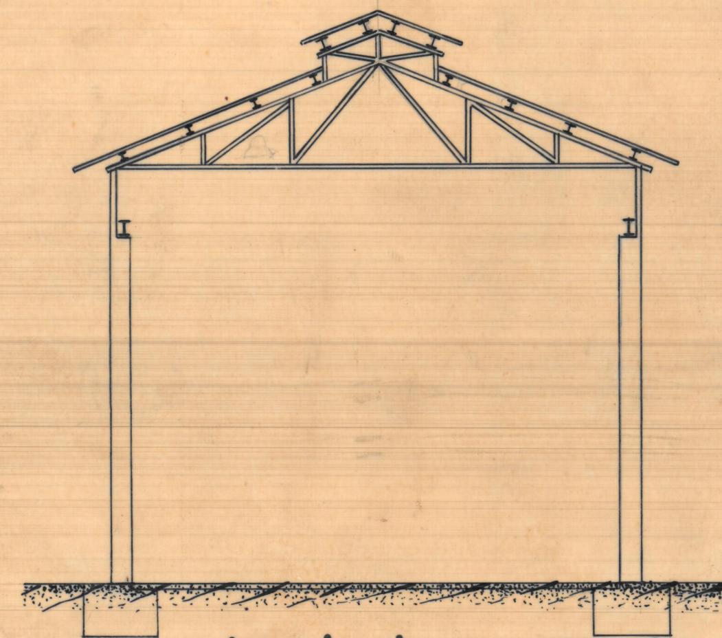
Alzado de la nave de fundición
