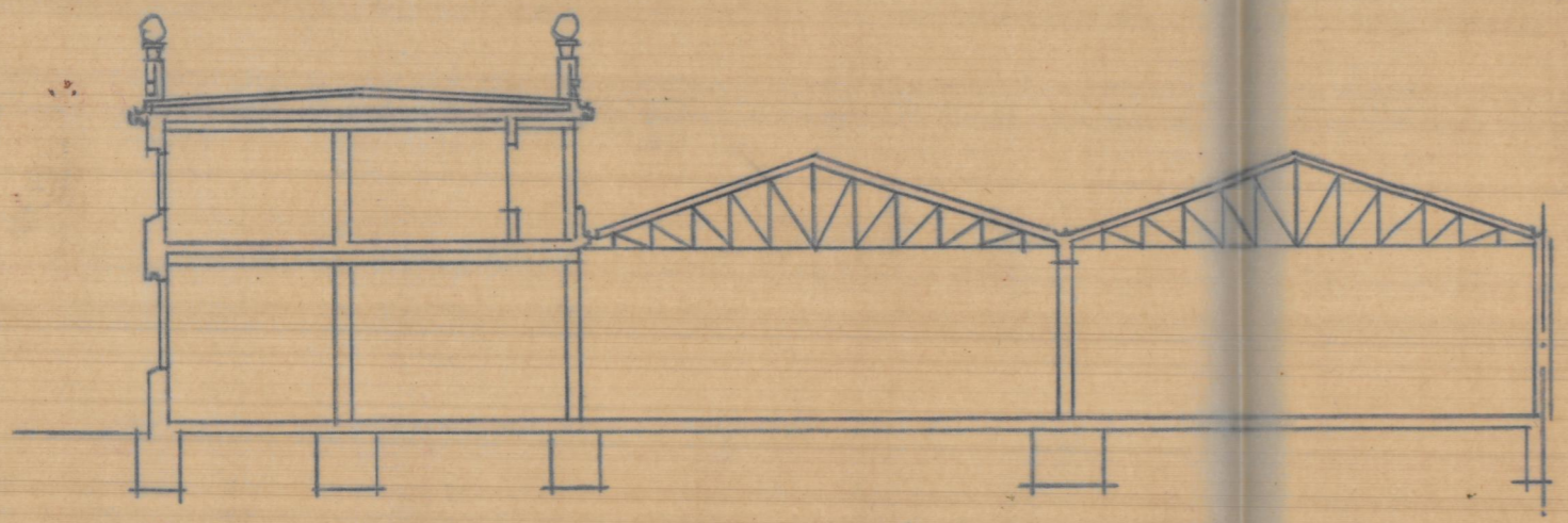
Seccion transversal
