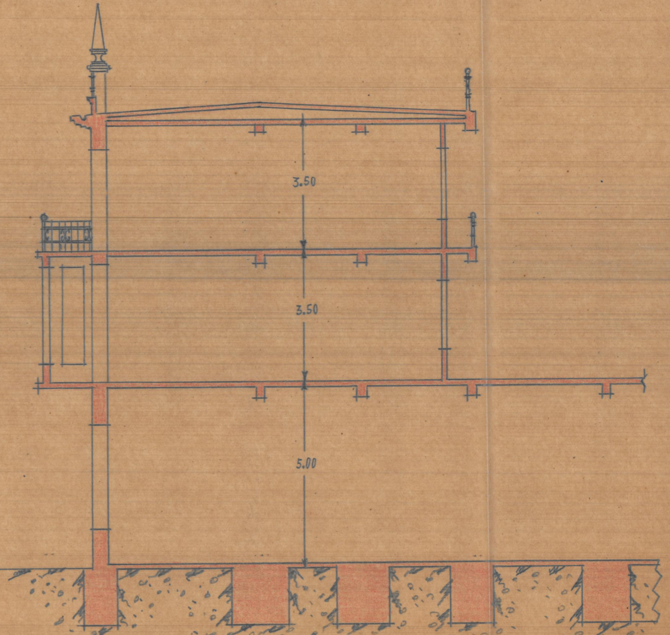
Sección por A-B
