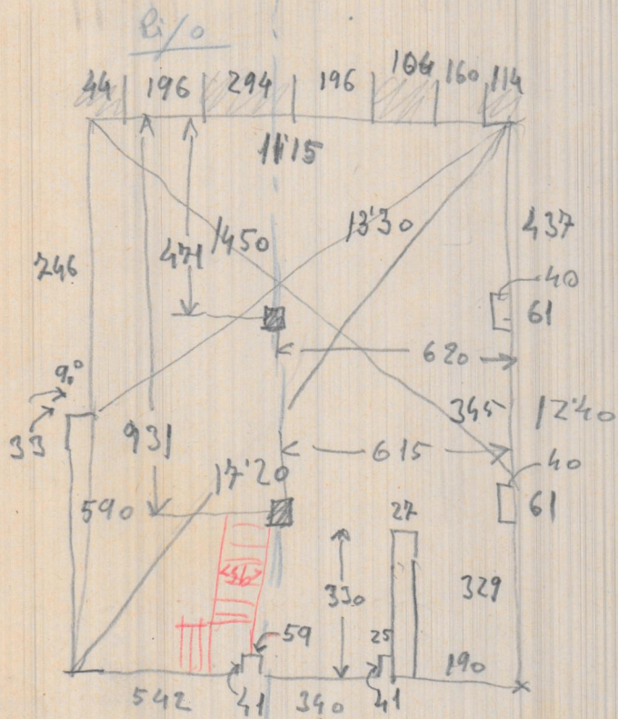
Seção Pilar 12
