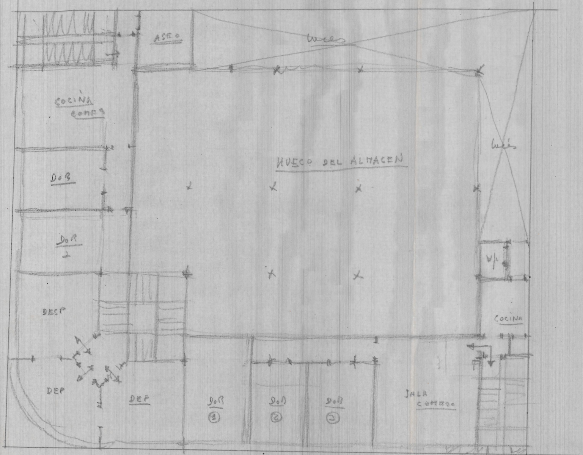
CALLE PLANTA DEL ENTREPISO
