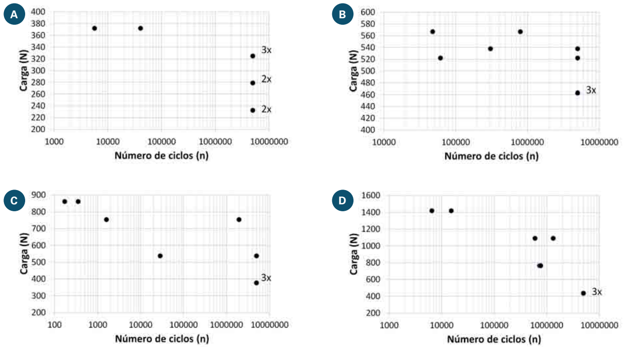
Figura 5. Diagramas de carga cíclica para cada modelo de pilar dental: (a) UCS33, (b) PZIM35, (c) CO41 y (d) PDINT.
