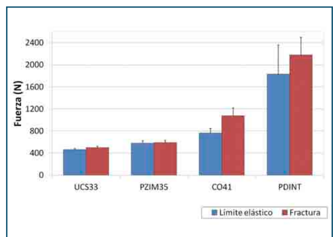
Figura 3. Resistencia estática de cada modelo de pilar dental.
