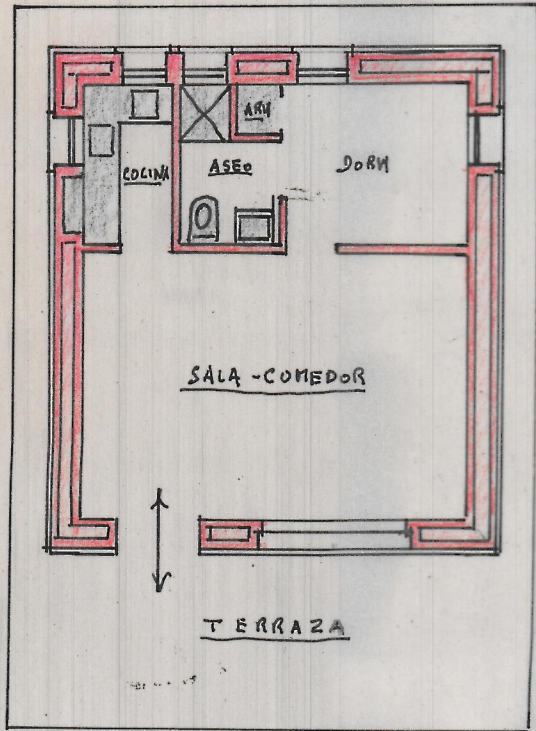
PLANTA DE DISTRIBUCION
