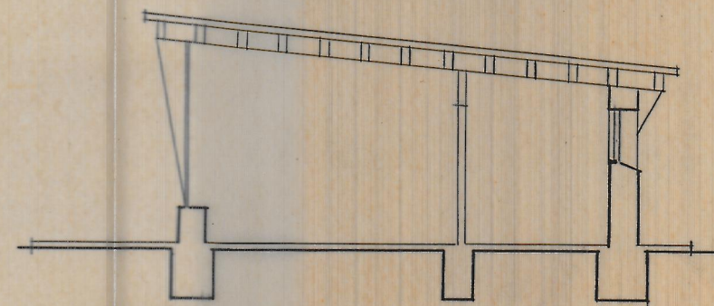
SECCION LONGITUDINAL
