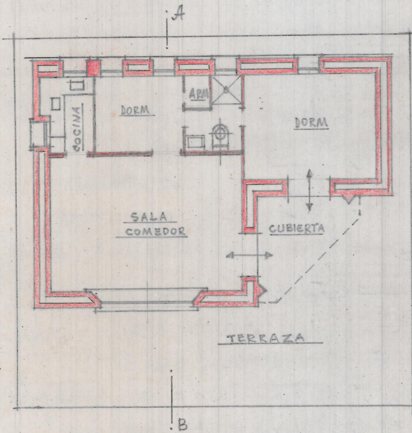
Planta de distribución
