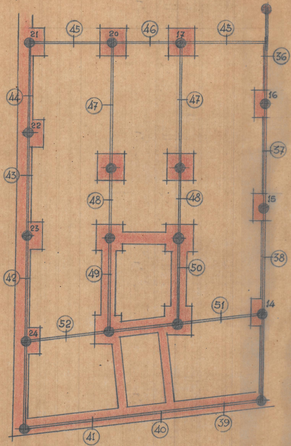
Planta de pilares, cimientos y entramado.
