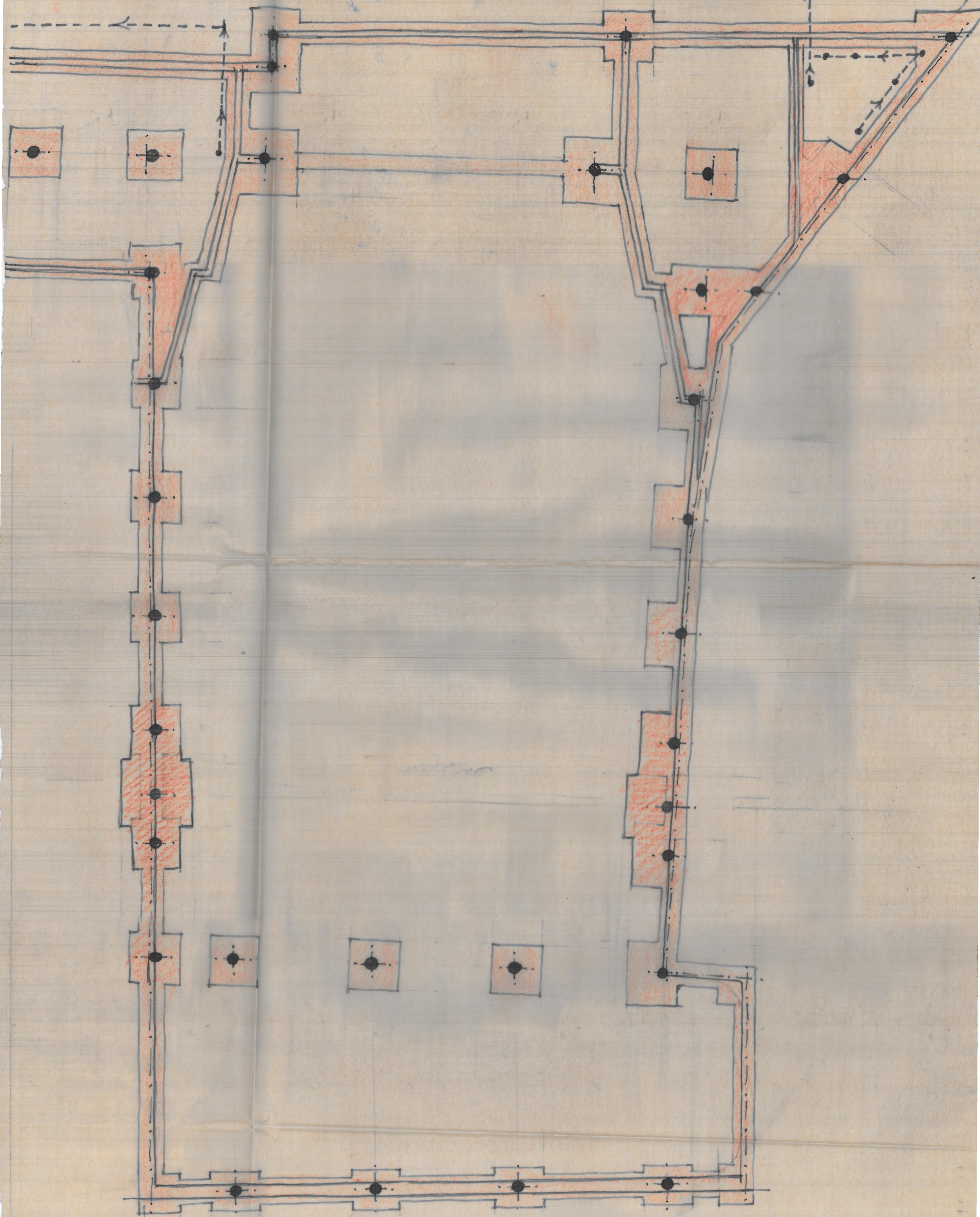
PLANTA DE CIMENTOS Y DESAGUES
