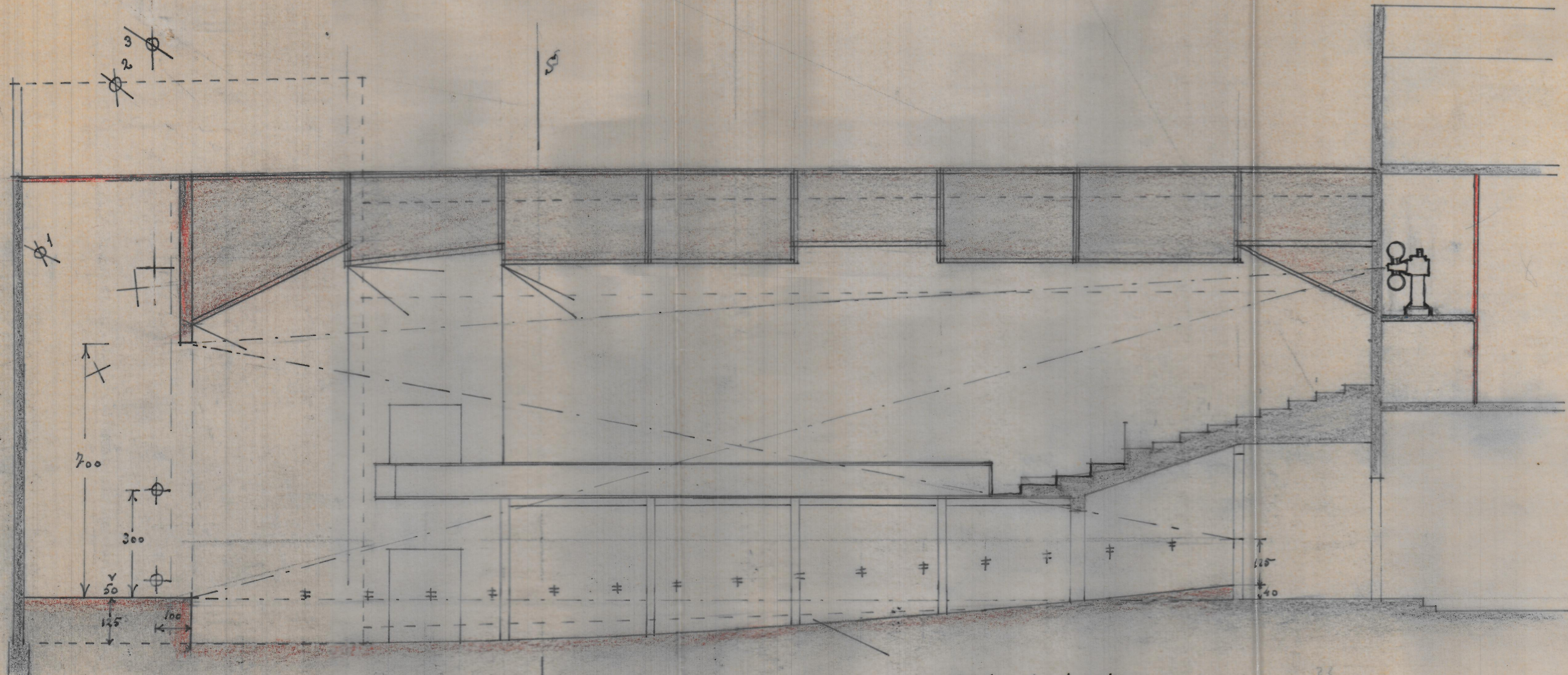
SECCION LONGITUDINAL
