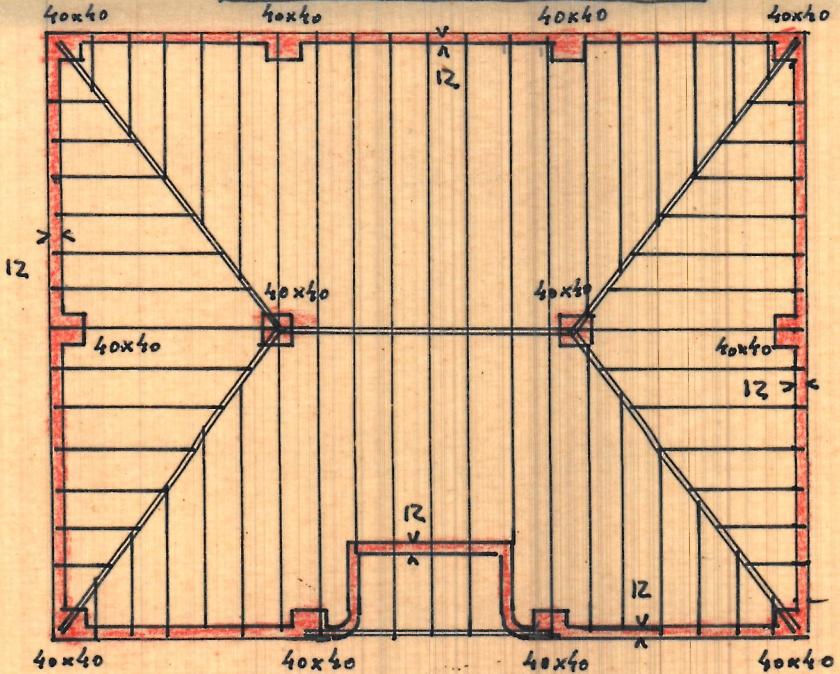
ESTRUCTURA DE CUBIERTA
