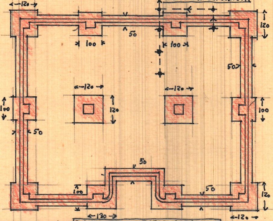
PLANTA DE CIMENTOS Y DESAGUES
