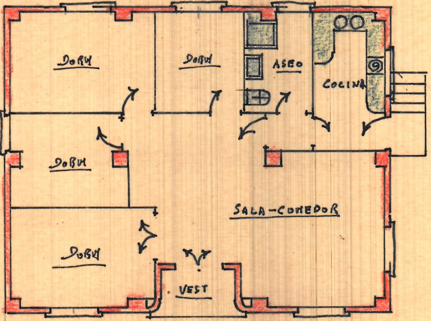
PLANTA DE DISPOSICION
