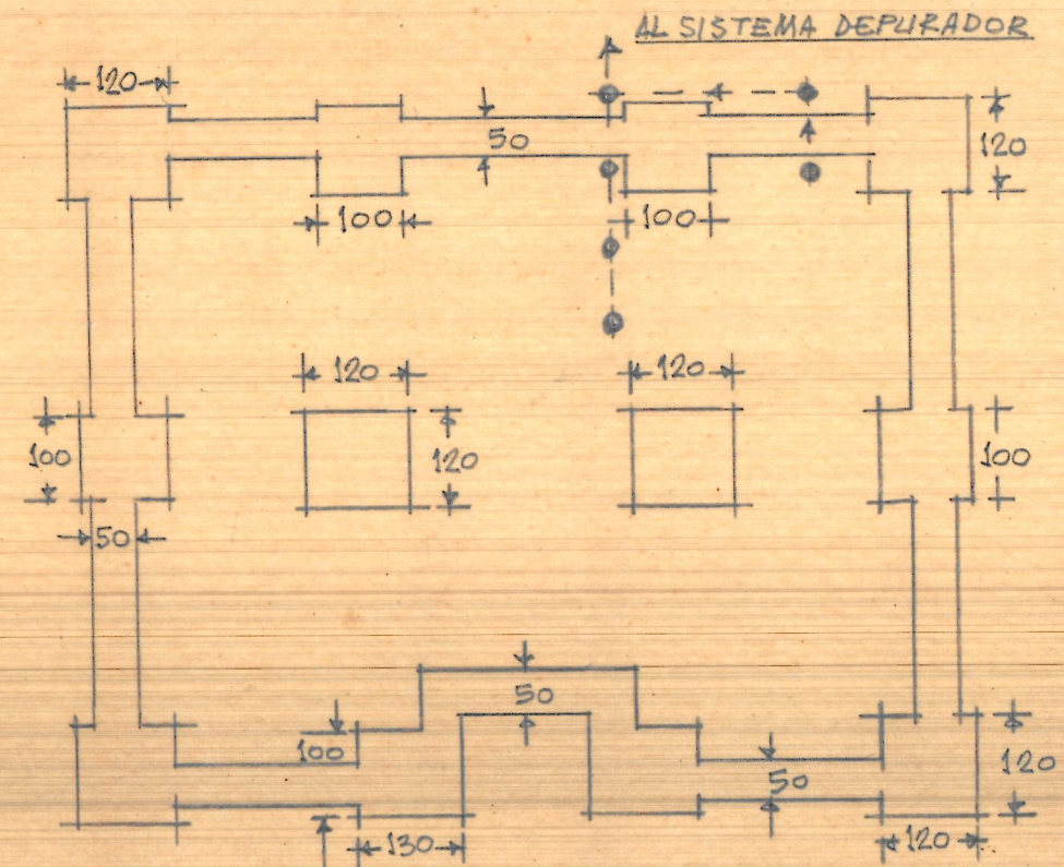
Plantas de alcantarillas y desagües
