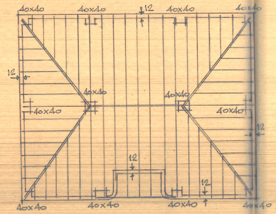
Estructura de cubierta
