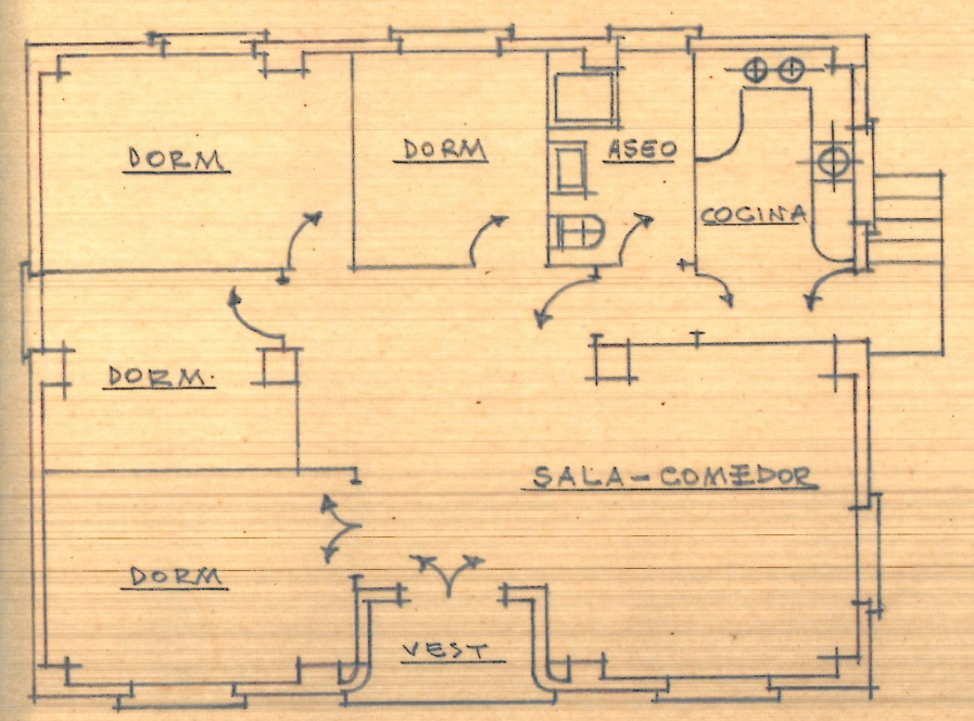
Plantas de distribución
