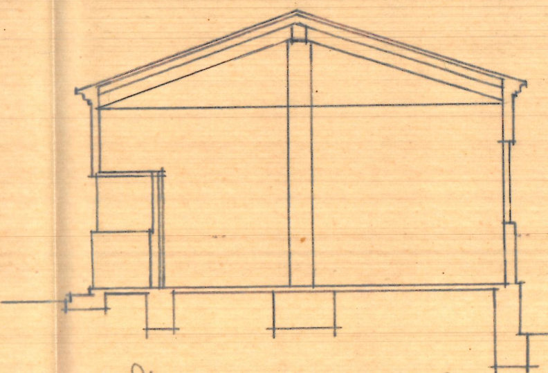
Sección por el eje
