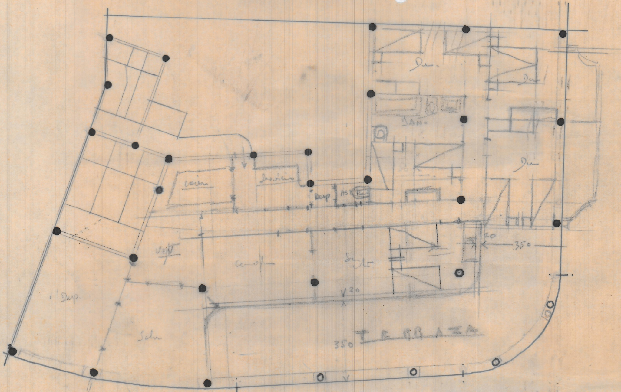
PLANTA DE ATICOS
