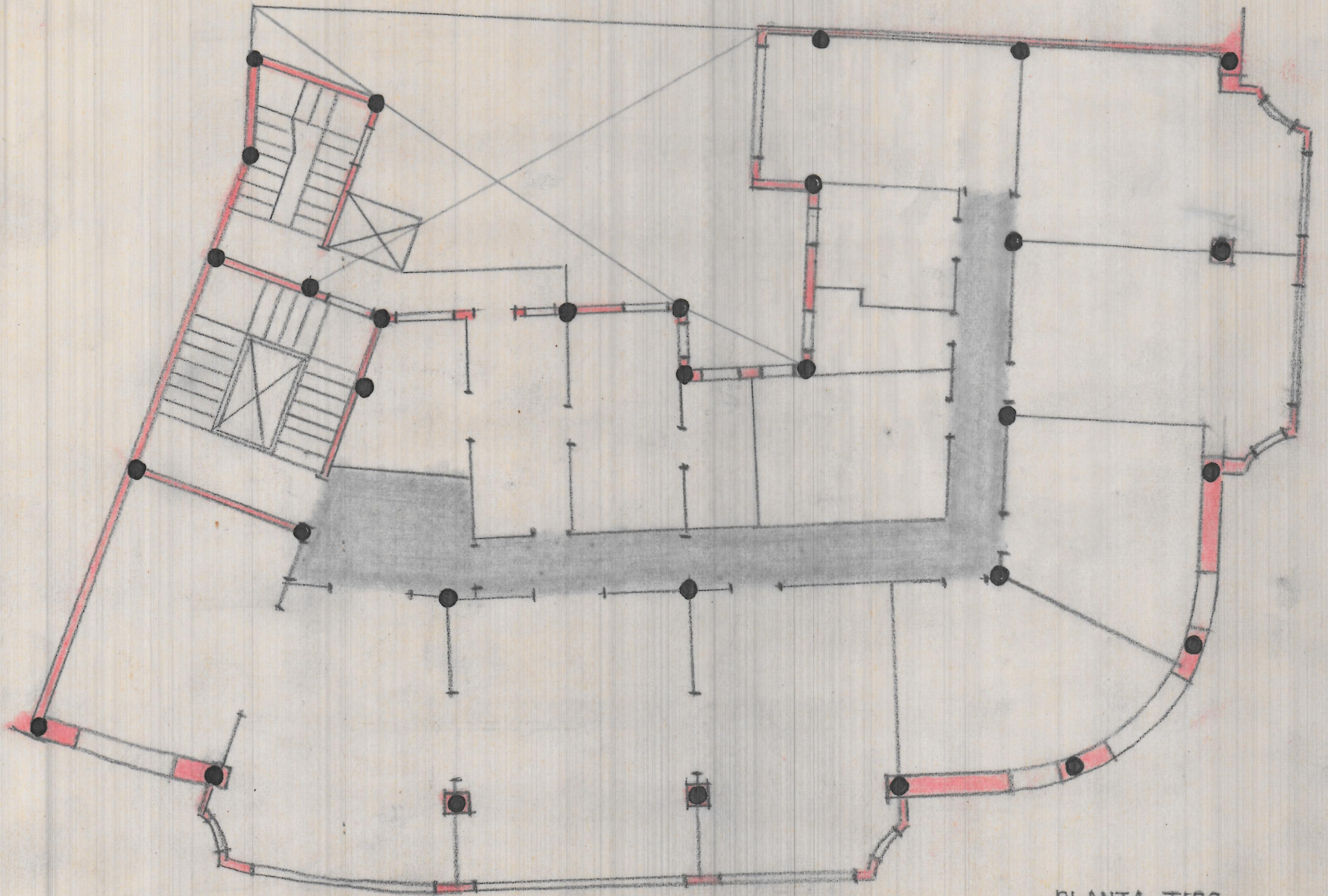
PLANTA TIPO E. I:100
