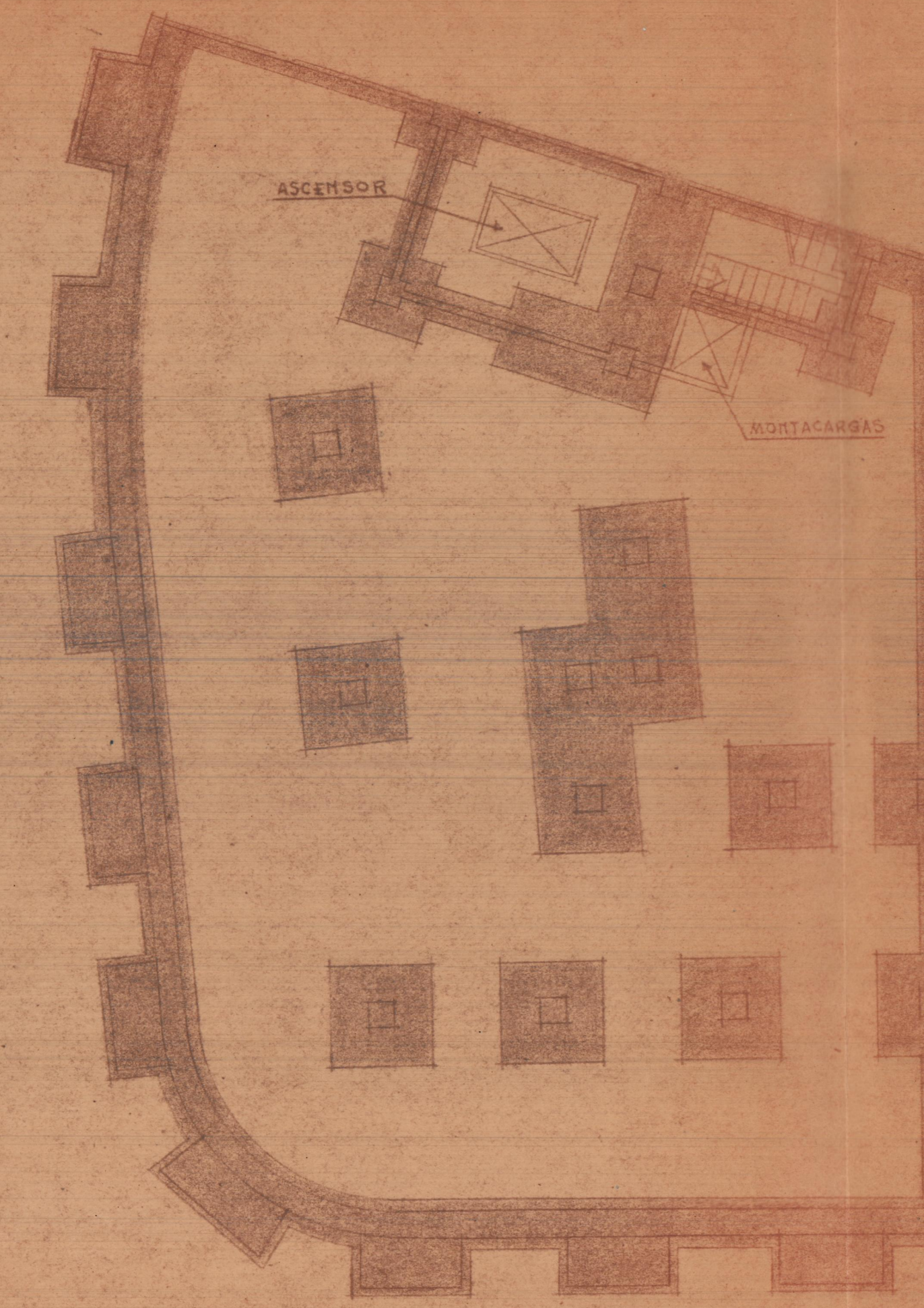
Planta de cimentación y solar
