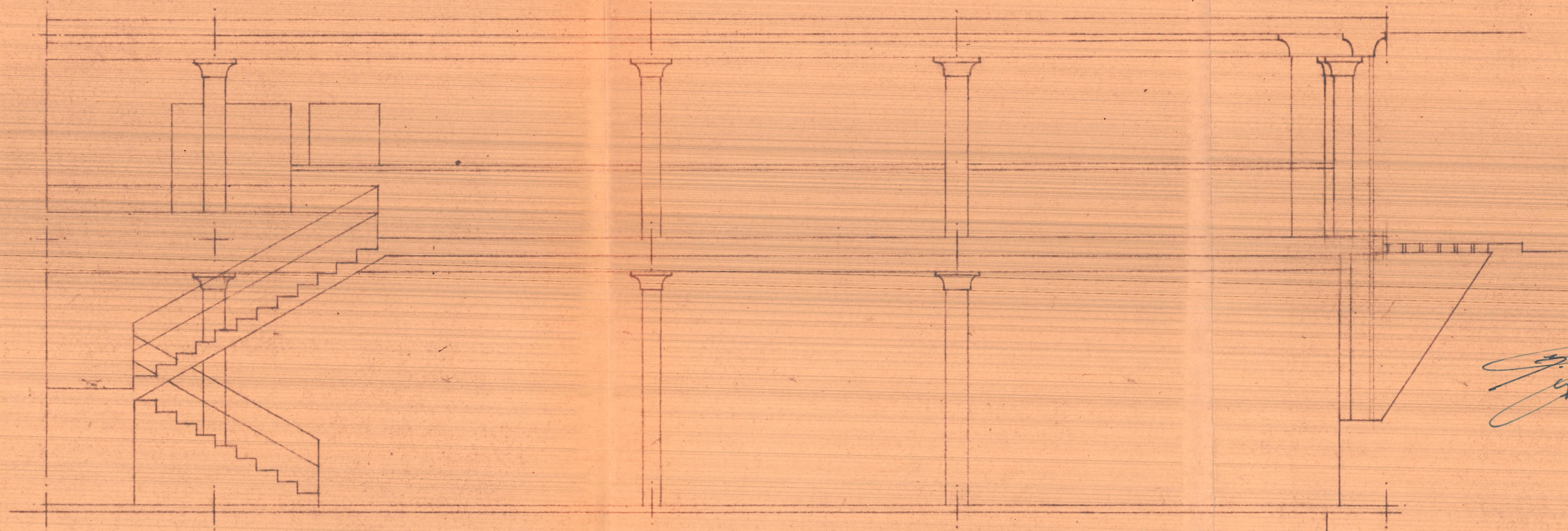
Sección longitudinal
